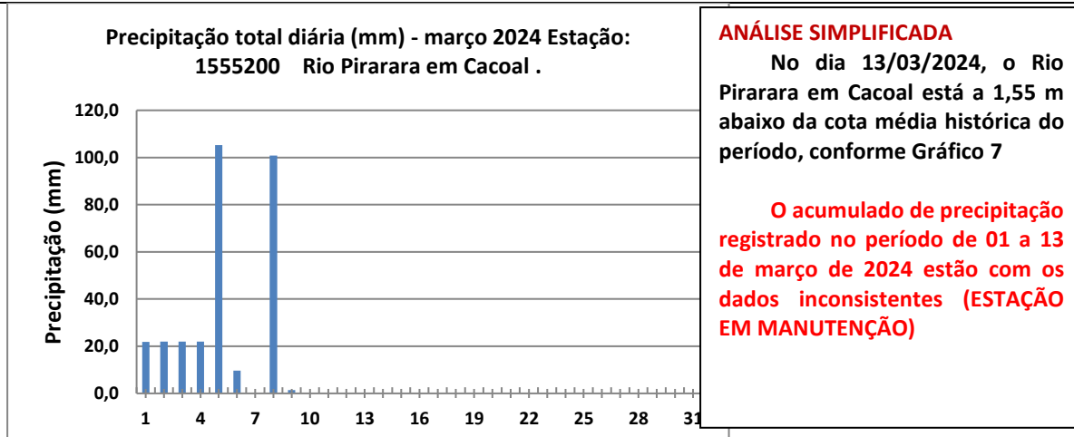
Gráfico 7.1 - Monitoramento da precipitação total diária, na estação meteorológica de Cacoal – código 01161008, no rio Pirara, em Cacoal - RO.
