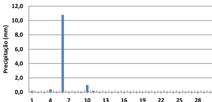
Gráfico 1.1- Monitoramento da precipitação total diária (mm), na estação pluviométrica Príncipe da Beira - código 01264000. Total mensal :
