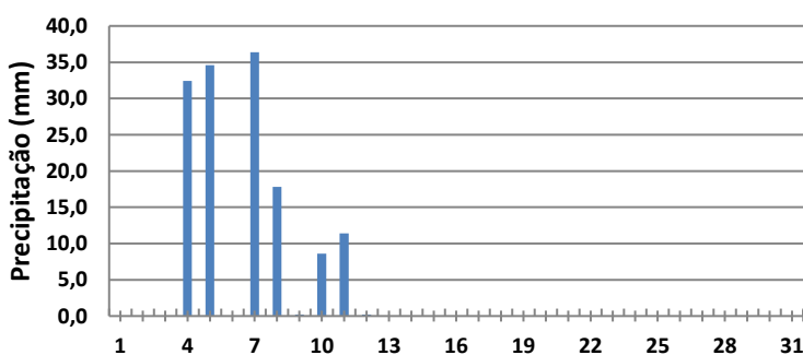
Rio Machado - Sítio Bela Vista em Pimenta Bueno Precipitação total diária (mm) - março 2024
