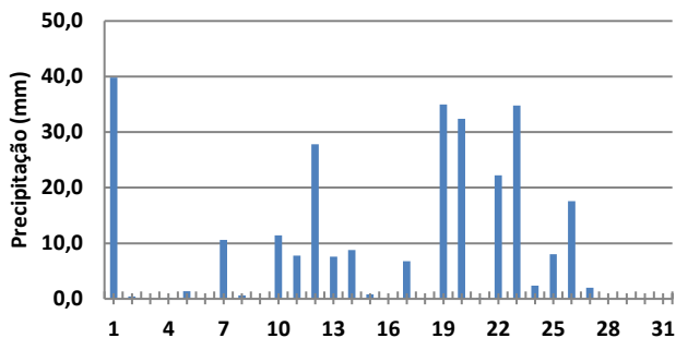
Precipitação total diária (mm) - fevereiro 2024 Estação 15560000 Rio Machado em Ji-Paraná .
