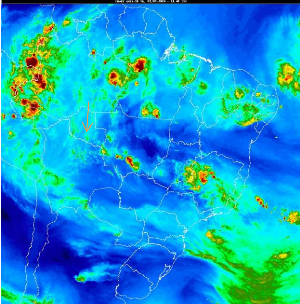
Fig. 1- Mapa da precipitação de 01/03/2024: satélite GOES, VA– 11:40 UTC Fonte: https://satelite.inmet.gov.br/N
