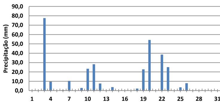
Precipitação total diária (mm) - fevereiro 2024. Rio Machado - Sítio Bela Vista em Pimenta Bueno .
