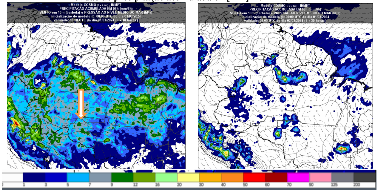
Figura 2 – Previsão do tempo no Estado de Rondônia para o dia 01/03/2024 as 18UTC
