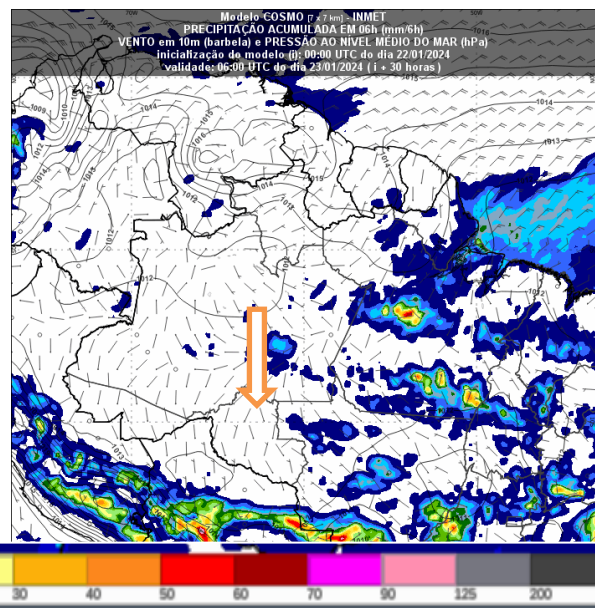
Figura 3 – Previsão do tempo no Estado de Rondônia para o dia 23/01/2024 às 06UTC
