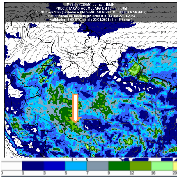
Figura 2 – Previsão do tempo no Estado de Rondônia para o dia 22/01/2024 às 18UTC
