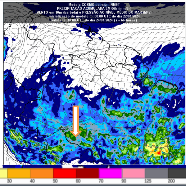
Figura 5 – Previsão de precipitação acumulada em RO, válida para 24/01/2024 18h
