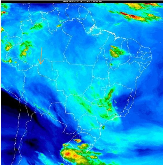
Fig. 1- Mapa da precipitação de 06/12/2023: satélite GOES, VA– 11:40 UTC Fonte: https://satelite.inmet.gov.br/N
