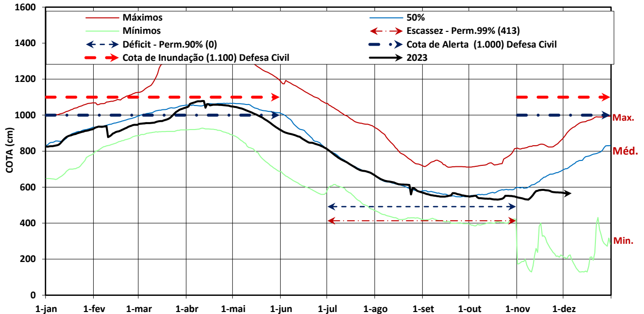
Gráfico 2- Monitoramento diário da cota do rio Mamoré, na coordenada geográfica de latitude 10,7925º leste e longitude 65,3478º oeste, município de Guajará-Mirim /RO - Série histórica 1970 a 2017.
