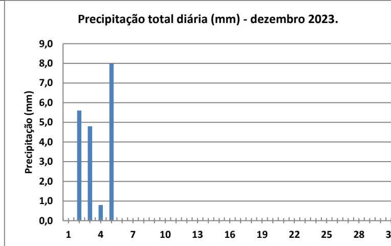
Gráfico 7.1 - Monitoramento da precipitação total diária, na estação meteorológica de Cacoal – código 01161008, no rio Pirarara, em Cacoal - RO. Fonte: organizado pela Sala de Situação - SEDAM com base nos dados disponíveis em: 1) http://mapas-hidro.ana.gov.br ; 2) http://sinda.crn2.inpe.br/PCD/SITE/novo/site/cidades.php?uf=RO ; 3) http://www.sedam.ro.gov.br/index.php/simego
