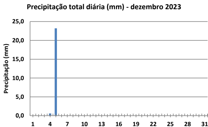
Gráfico6.1- Monitoramento da precipitação total diária, na estação meteorológica Ji-Paraná – código 1061001, no rio Machado, em Ji-Paraná - RO.
