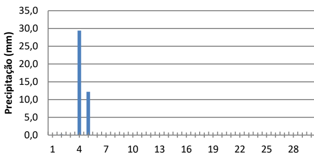
Precipitação total diária (mm) - Dezembro 2023 Estação: 15250000 GUAJARÁ-MIRIM
