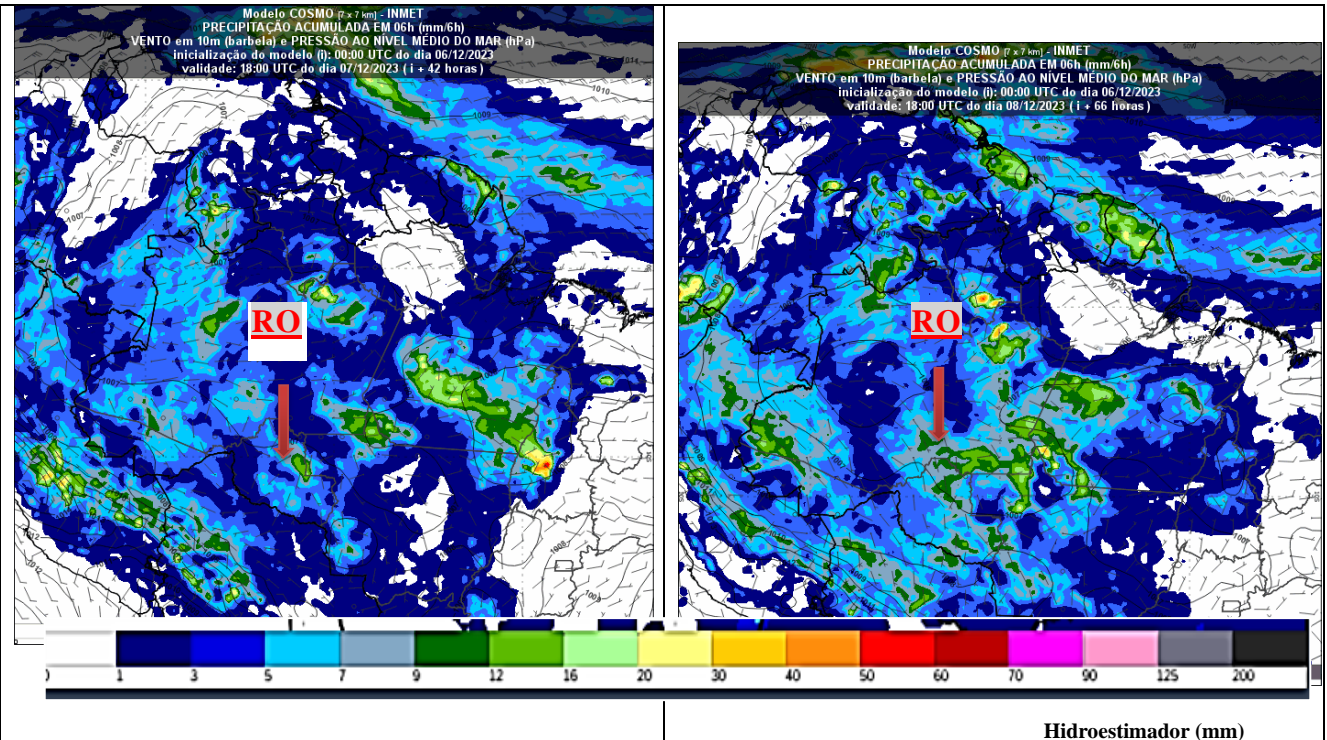
Figura 4 – Previsão de precipitação acumulada em RO, válida para 07/12/2023 8h Fonte: http://www.inmet.gov.br/
