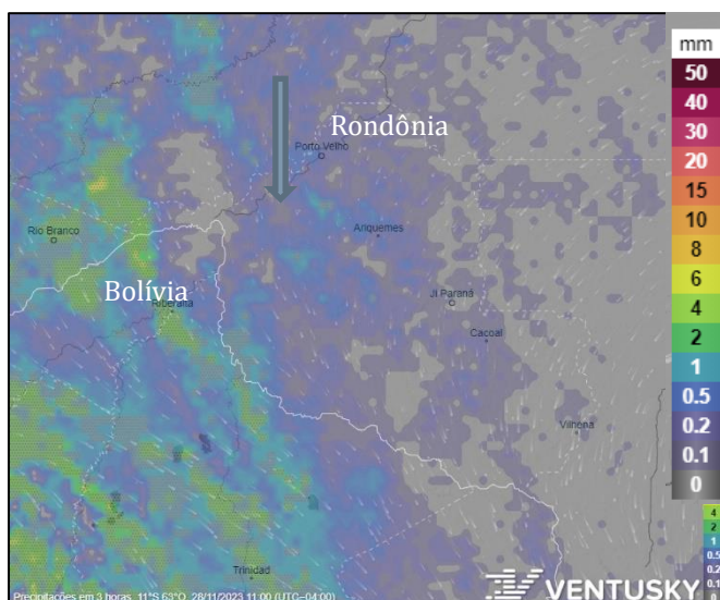
Figura 2 – Precipitação registrado as 11h 28/11/2023 Dados de satélite
