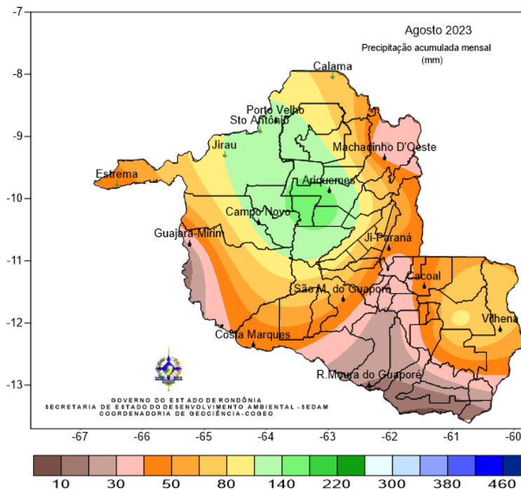
Figura 2 - Mapa da precipitação acumulada em agosto de 2023, com base nos dados da SEDAM/RO, ANA e INMET
