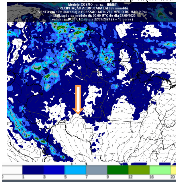
Figura 2 – Previsão do tempo no Estado de Rondônia para o dia 22/09/2023 as 18UTC
