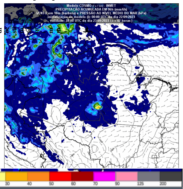
Figura 3 – Previsão do tempo no Estado de Rondônia para o dia 23/09/2023 as 06 UTC
