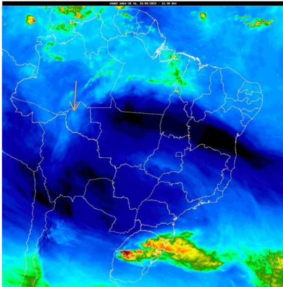
Fig. 1- Mapa da precipitação de 22/09/2023: satélite GOES, VA– 11:40 UTC Fonte: https://satelite.inmet.gov.br/N
