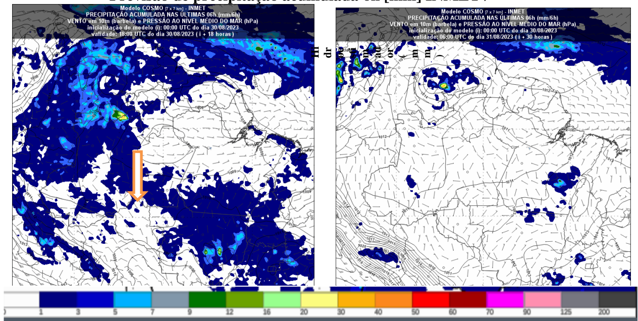
Figura 2 – Previsão do tempo no Estado de Rondônia para o dia 30/08/2023 as 18UTC
