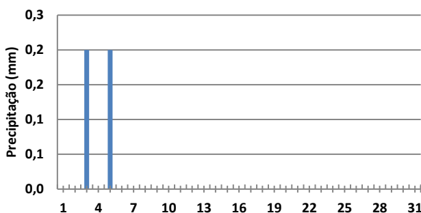
Precipitação total diária (mm) - julho 2023 Estação 15560000 Rio Machado em Ji-Paraná .
