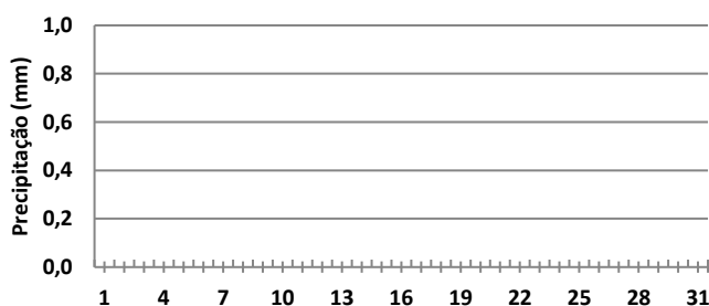
Precipitação total diária (mm) - julho 2023. 15400000 - Rio Madeira em Porto Velho
