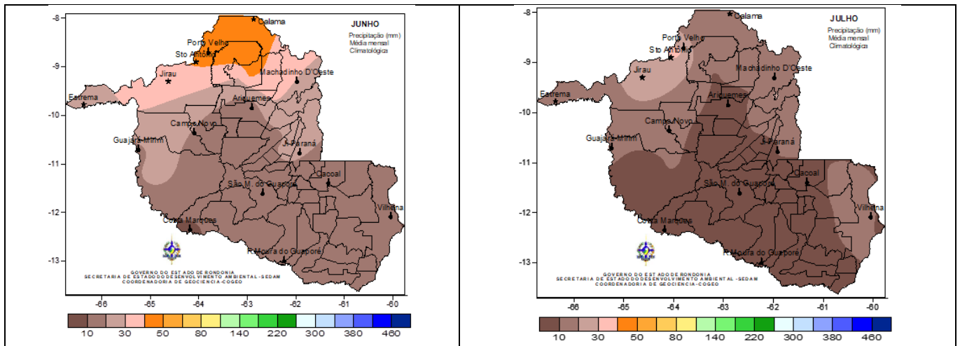
Fig. A- Climatologia de precipitação mensal, baseada nos métodos dos Quantis - 1970 a 2011. Fonte: Atualização da base do ZSEE-RO.
