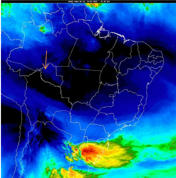
Fig. 1- Mapa da precipitação de 12/07/2023: satélite GOES, VA– 11:40 UTC Fonte: https://satelite.inmet.gov.br/N
