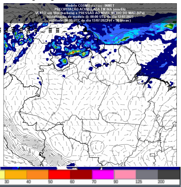
Figura 3 – Previsão do tempo no Estado de Rondônia para o dia 13/07/2023 as 06 UTC
