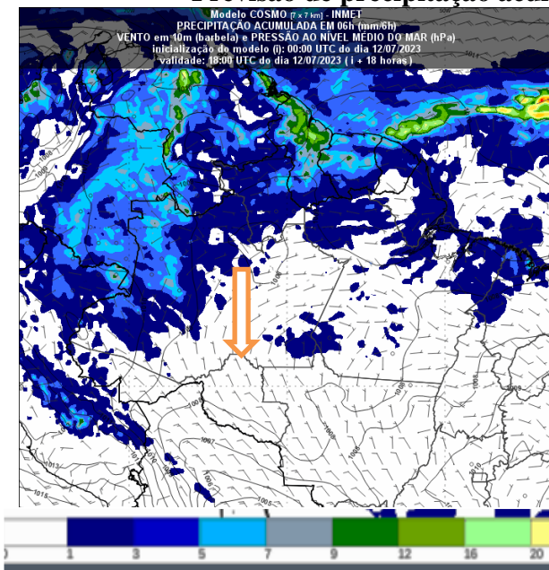
Figura 2 – Previsão do tempo no Estado de Rondônia para o dia 12/07/2023 as 18UTC
