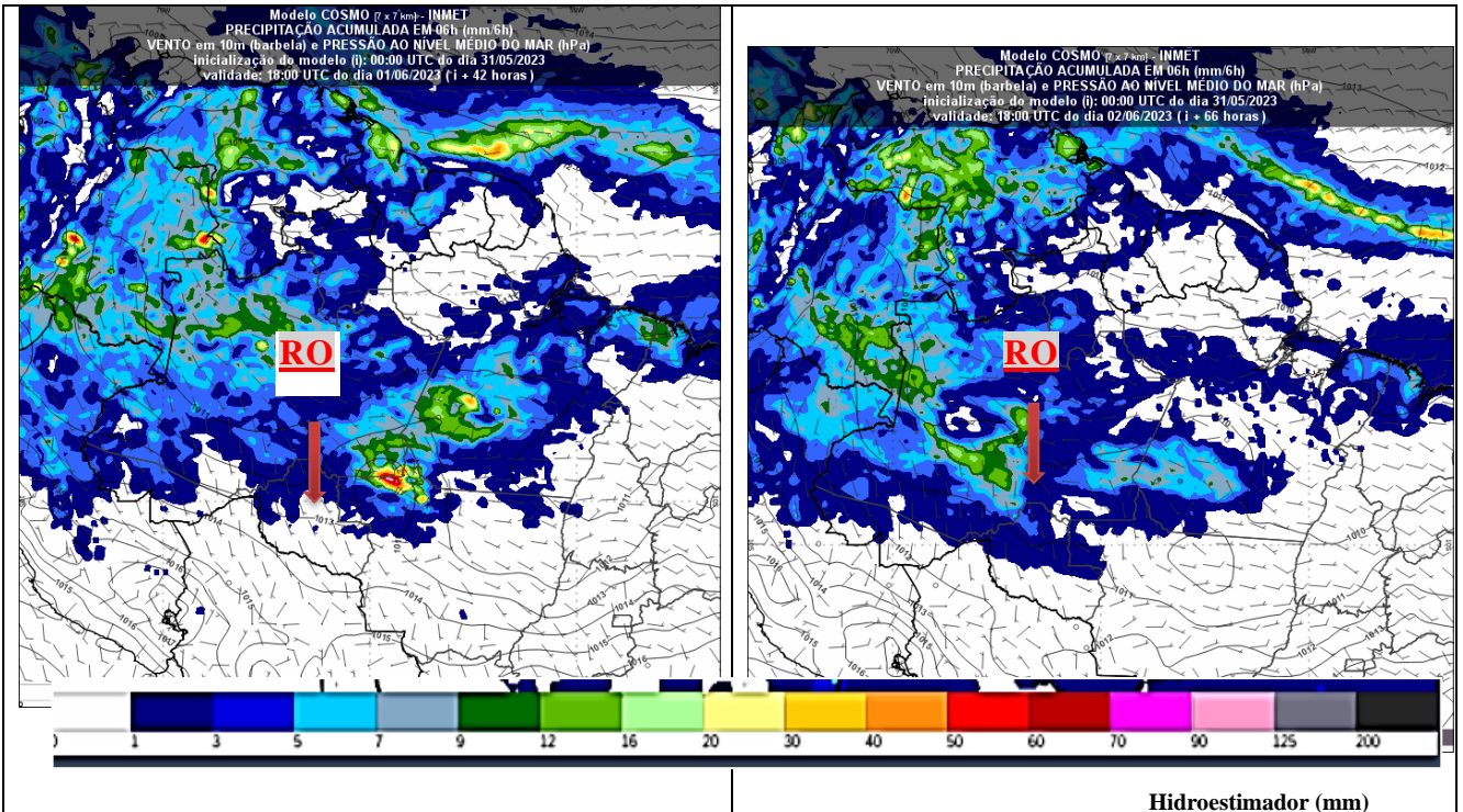
Figura 4 – Previsão de precipitação acumulada em RO, válida para 01/06/2023 8h Fonte: http://www.inmet.gov.br/
