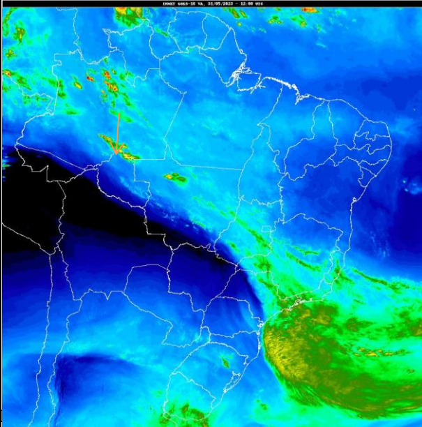
Figura 1 – satélite GOES, VA 31/05/2023 – 11:40 UTC Fonte: https://satelite.inmet.gov.br/N
