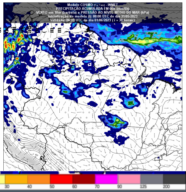
Figura 3 – Previsão do tempo no Estado de Rondônia para o dia 01/06/2023 as 06 UTC
