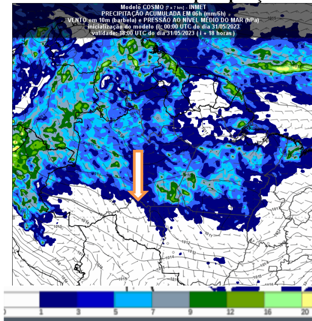
Figura 2 – Previsão do tempo no Estado de Rondônia para o dia 31/05/2023 as 18UTC
