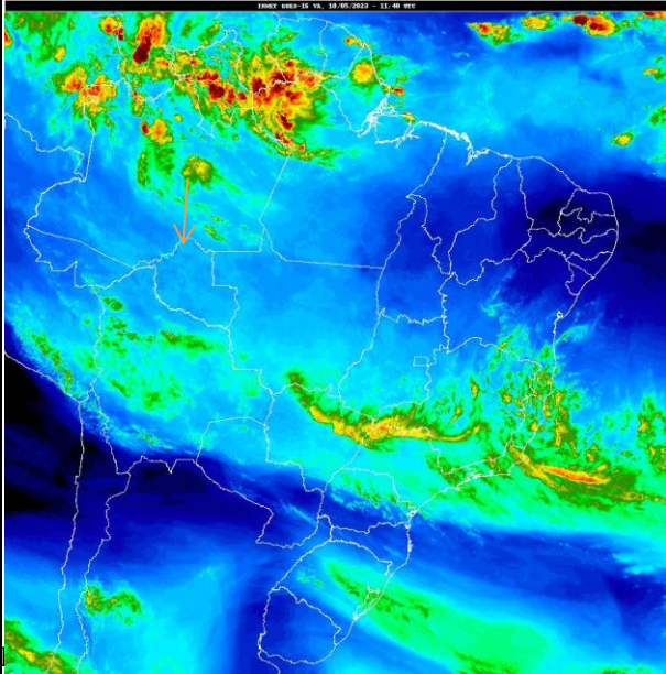
Figura 1 – satélite GOES, VA 10/05/2023 – 11:40 UTC Fonte: https://satelite.inmet.gov.br/N
