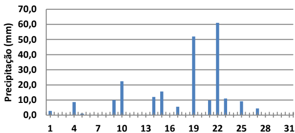
Precipitação total diária (mm) - Abril 2023. Estação 15560000 Rio Machado em Ji-Paraná
