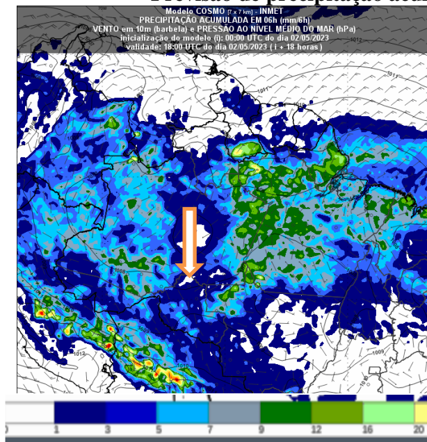
Figura 2 – Previsão do tempo no Estado de Rondônia para o dia 02/05/2023 as 18UTC
