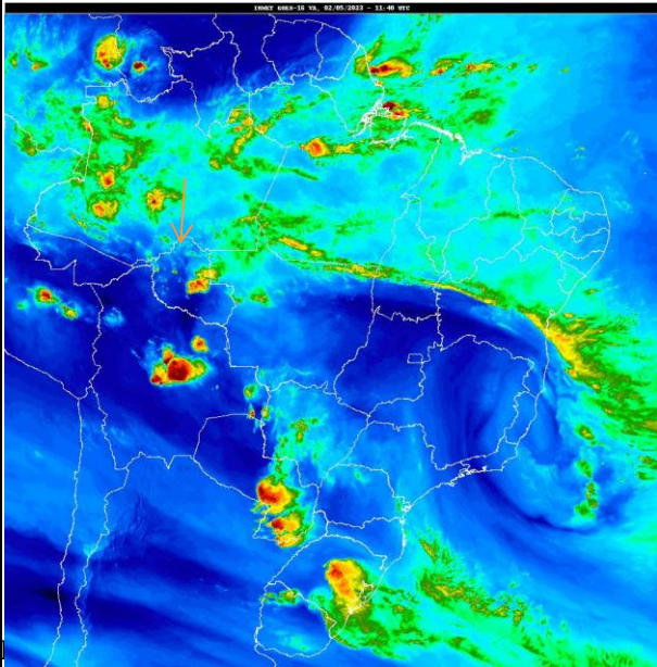
Figura 1 – satélite GOES, VA 02/05/2023 – 11:40 UTC Fonte: https://satelite.inmet.gov.br/N
