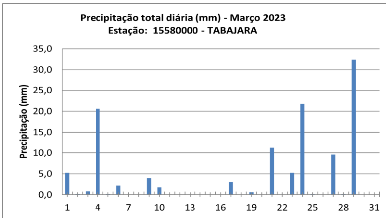
Gráfico 2 - Precipitação total diária na estação Pluviométrica próximo a Machadinho do Oeste.
