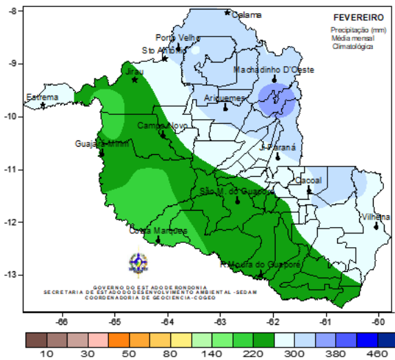
Figura 4 -. Climatologia de precipitação mensal , baseada no métodos dos Quantis - 1970 a 2011 (fevereiro)
