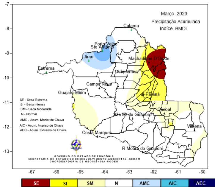
Figura 3 - Classificação da precipitação acumulada pelo Índice BMDI em março de 2023, com base nos dados do ZEE/RO, SEDAM/RO, ANA e INMET.
