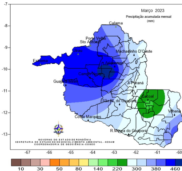
Figura 2 - Mapa da precipitação acumulada em março de 2023, com base nos dados da SEDAM/RO, ANA e INMET
