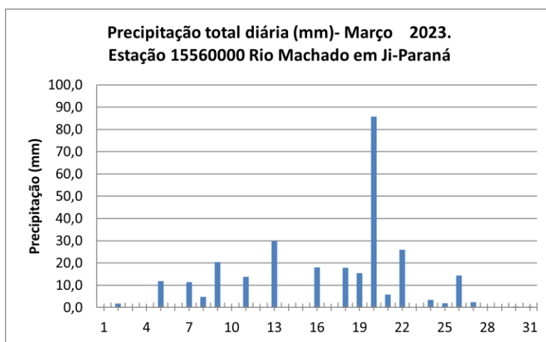
Gráfico 1 - Precipitação total diária na estação Pluviométrica em Ji-Paraná.
