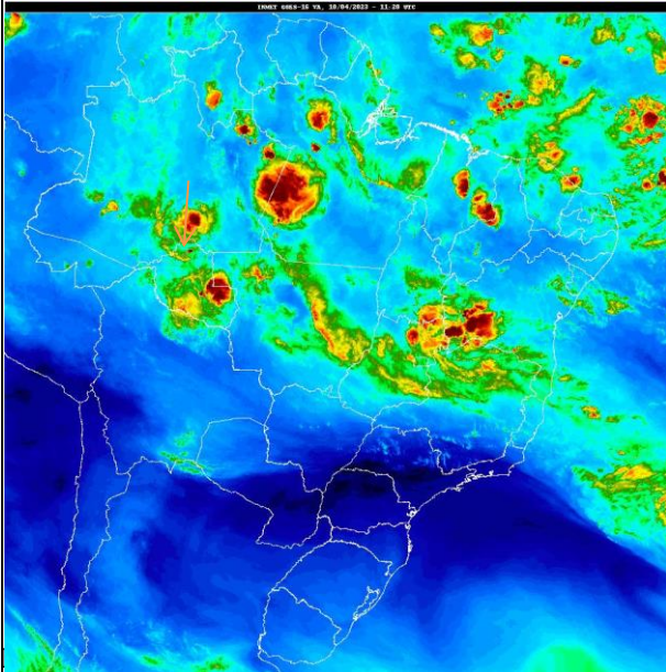
Figura 1 – satélite GOES, VA 10/04/2023 – 11:40 UTC Fonte: https://satelite.inmet.gov.br/N
