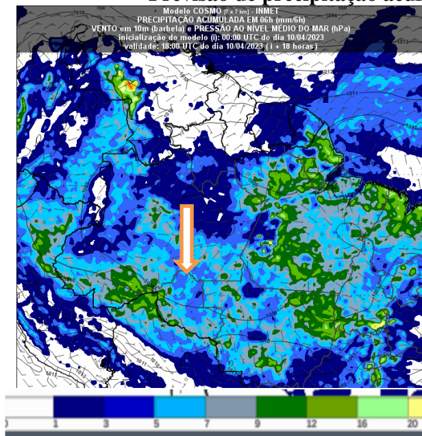
Figura 2 – Previsão do tempo no Estado de Rondônia para o dia 10/04/2023 as 18UTC
