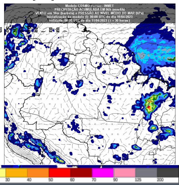
Figura 3 – Previsão do tempo no Estado de Rondônia para o dia 11/04/2023 as 06 UTC
