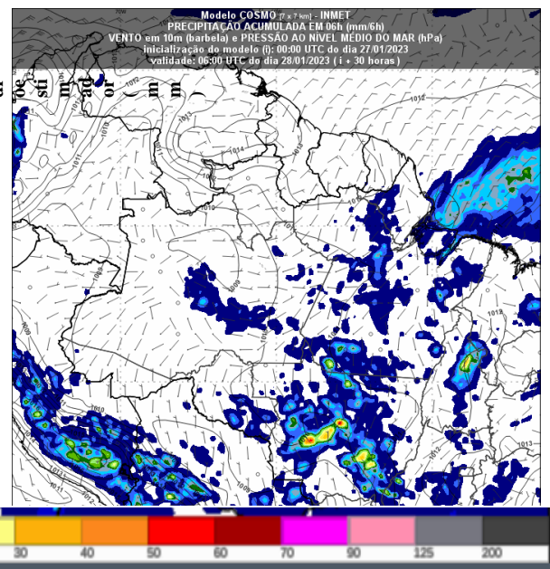
Figura 3 – Previsão do tempo no Estado de Rondônia para o dia 28/01/2023 as 06 UTC
