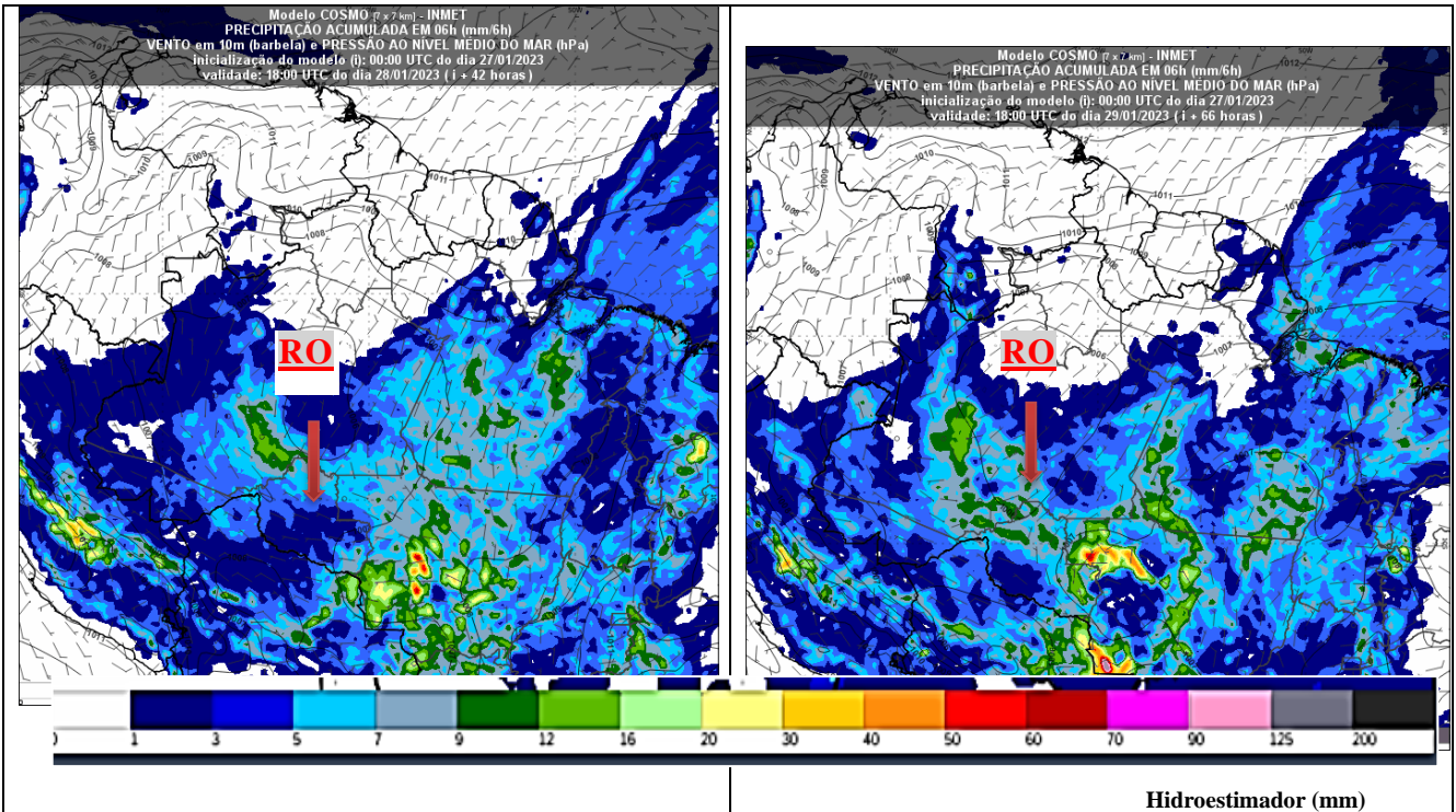
Figura 4 – Previsão de precipitação acumulada em RO, válida para 29/01/2023 8h Fonte: http://www.inmet.gov.br/
