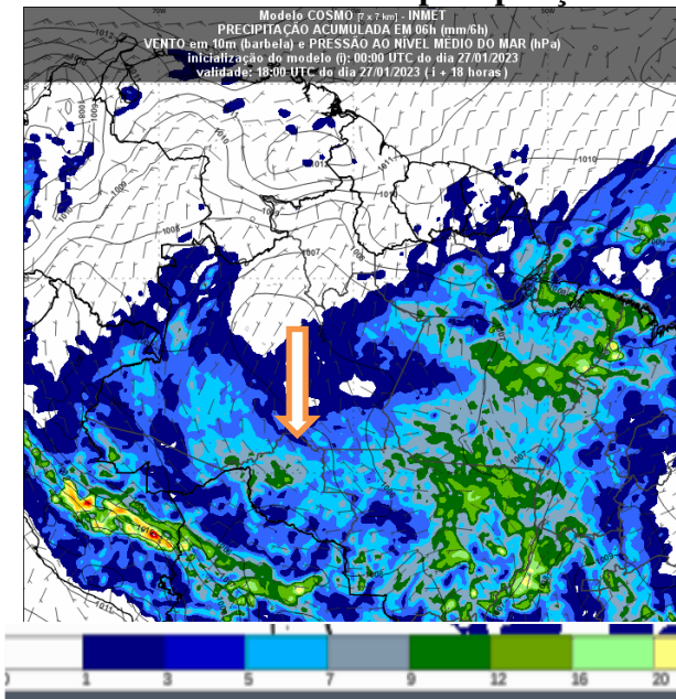
Figura 2 – Previsão do tempo no Estado de Rondônia para o dia 27/01/2023 as 18UTC
