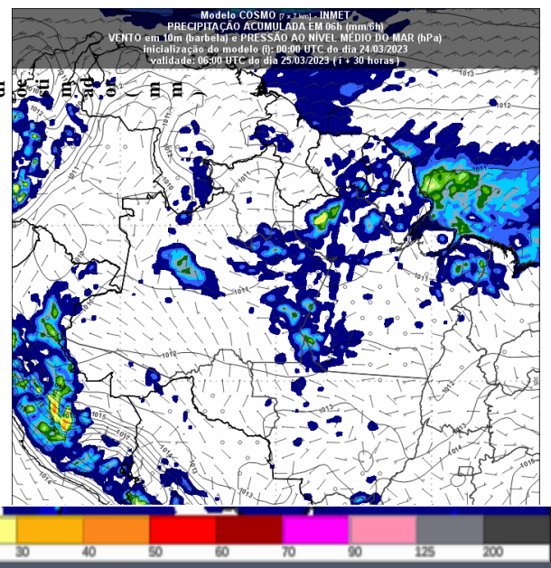
Figura 3 – Previsão do tempo no Estado de Rondônia para o dia 25/03/2023 as 06 UTC
