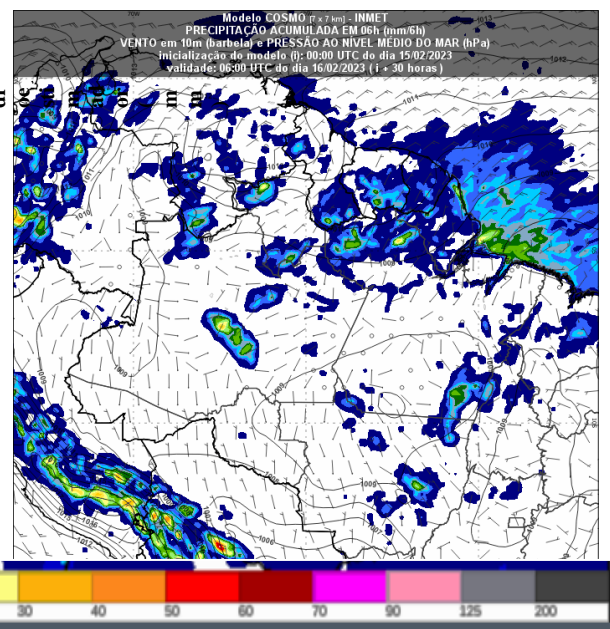
Figura 3 – Previsão do tempo no Estado de Rondônia para o dia 16/02/2023 as 06 UTC
