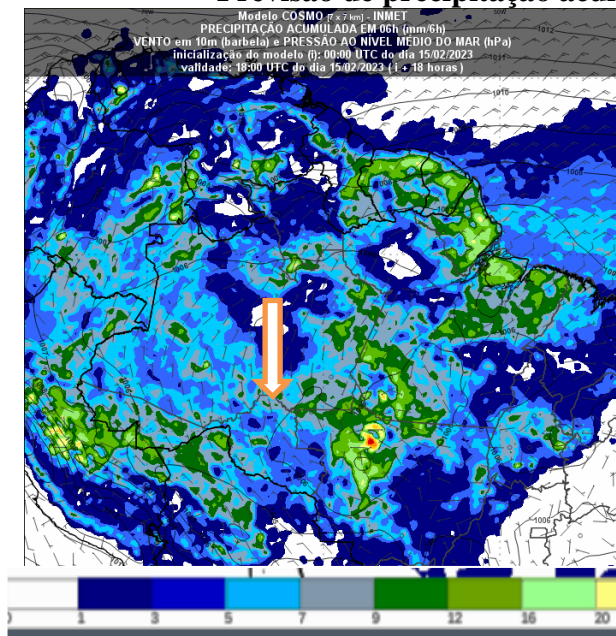
Figura 2 – Previsão do tempo no Estado de Rondônia para o dia 15/02/2023 as 18UTC
