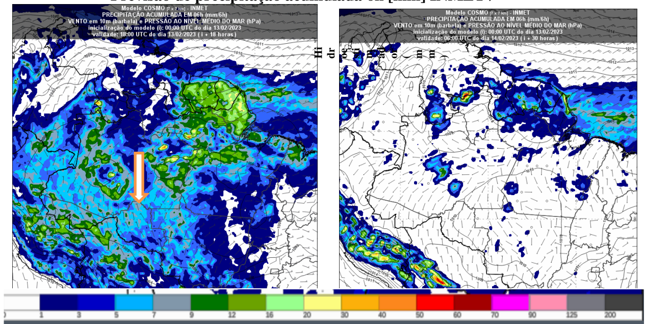
Figura 2 – Previsão do tempo no Estado de Rondônia para o dia 13/02/2023 as 18UTC
