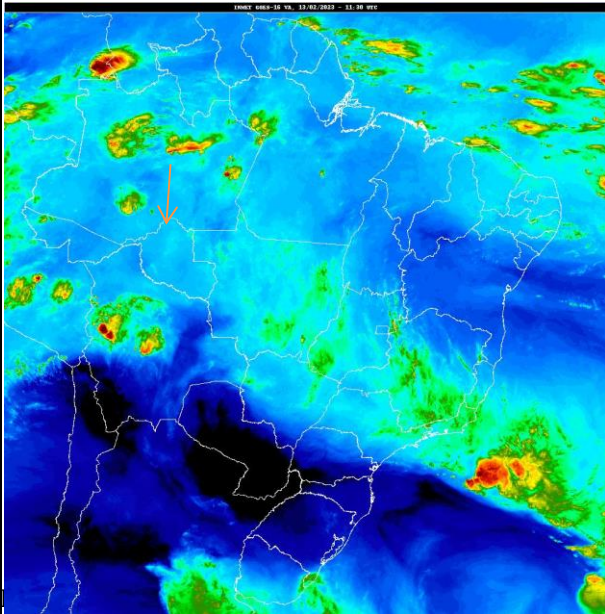
Figura 1 – satélite GOES, VA 13/02/2023 – 11:40 UTC Fonte: https://satelite.inmet.gov.br/N
