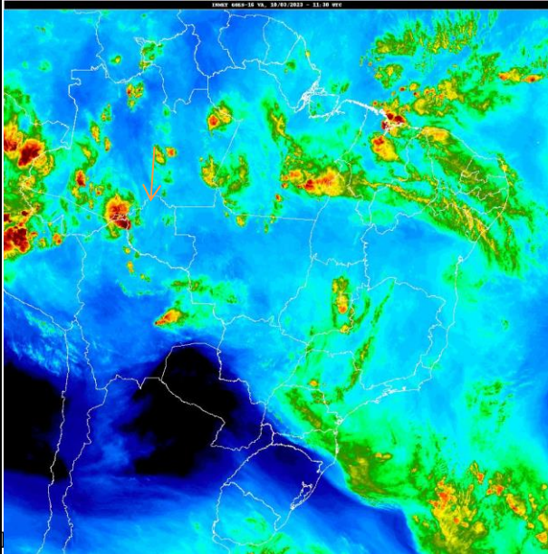
Figura 1 – satélite GOES, VA 10/03/2023 – 11:40 UTC Fonte: https://satelite.inmet.gov.br/N
