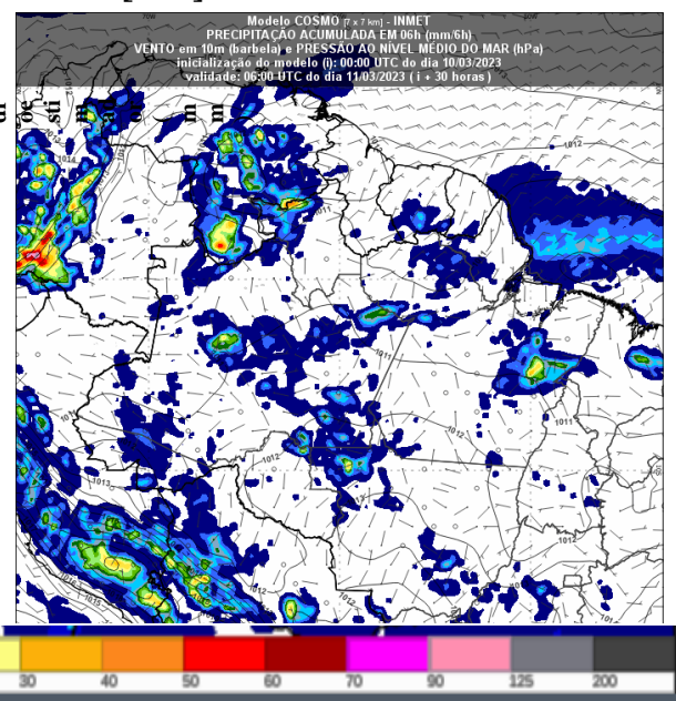
Figura 3 – Previsão do tempo no Estado de Rondônia para o dia 11/03/2023 as 06 UTC
