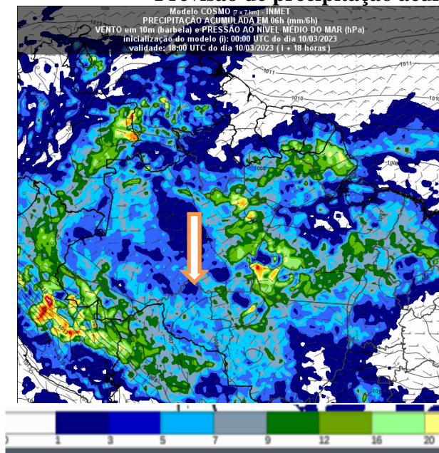
Figura 2 – Previsão do tempo no Estado de Rondônia para o dia 10/03/2023 as 18UTC
