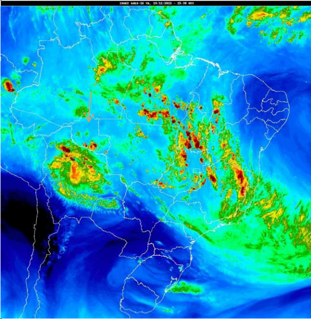
Fig. 1- Mapa da precipitação de 19/12/2022: Fonte: http://satellite.cptec.inpe.br/home/index.jsp
