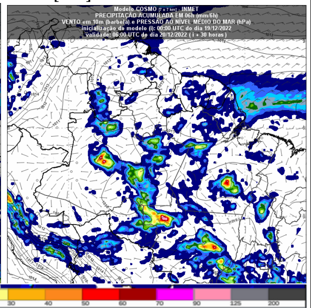
Figura 3 – Previsão do tempo no Estado de Rondônia para o dia 20/12/2022 as 06 UTC
