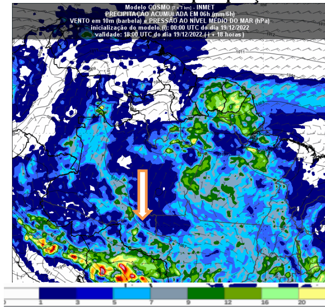
Figura 2 – Previsão do tempo no Estado de Rondônia para o dia 19/12/2022 as 18UTC
