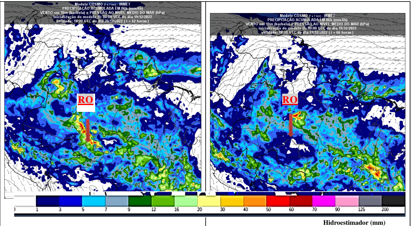
Figura 4 – Previsão de precipitação acumulada em RO, válida para 20/12/2022 18h
