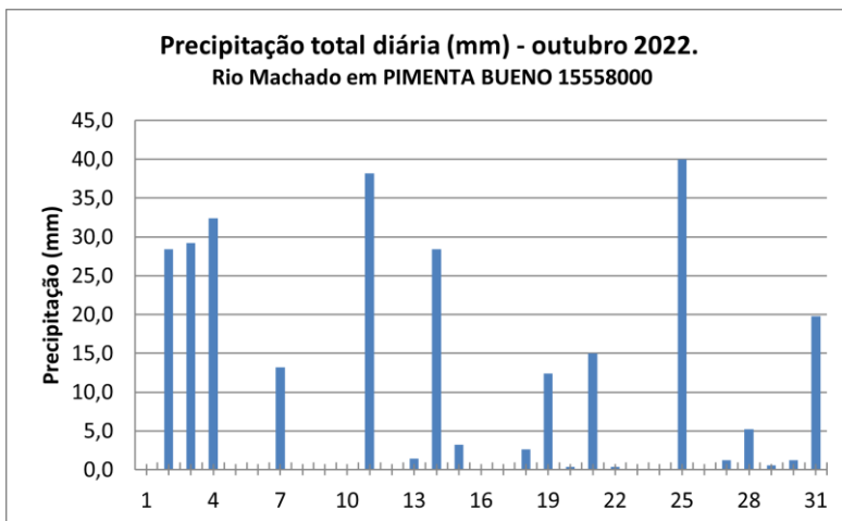
Gráfico 3 - Precipitação total diária na estação Pluviométrica em Pimenta Bueno.
