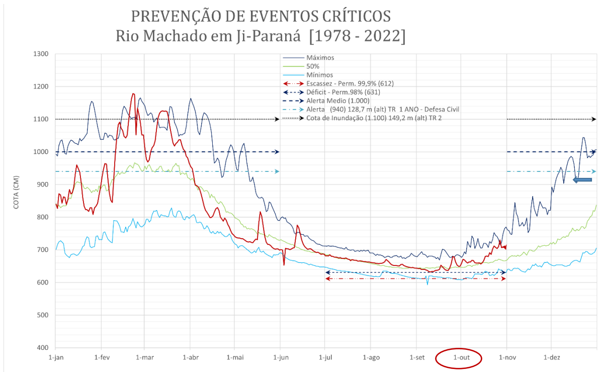
Gráfico 5 - Monitoramento diária de curva de permanência, com base nos dados da estação hidrológica de Ji-Paraná - código 15560000:
