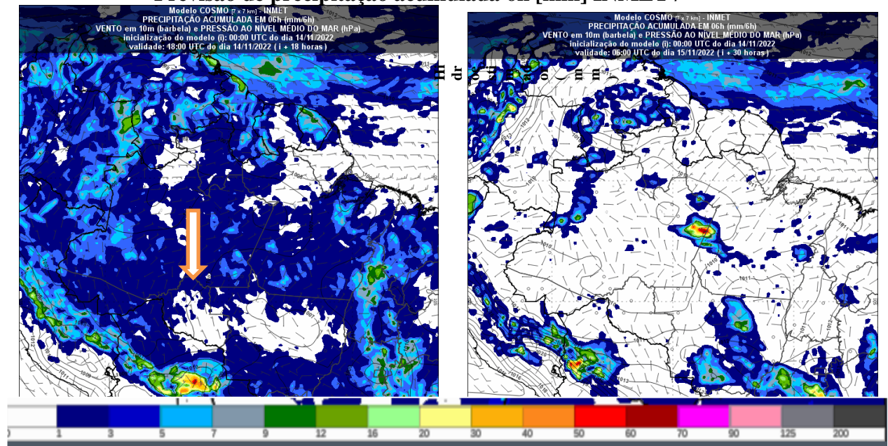
Figura 2 – Previsão do tempo no Estado de Rondônia para o dia 14/11/2022 as 18UTC
