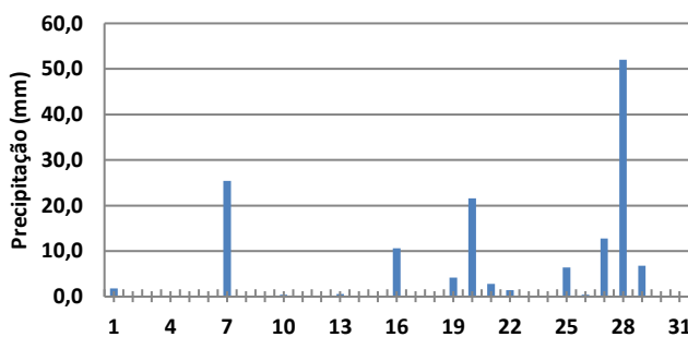
Precipitação total diária (mm) - outubro 2022 Estação 15560000 Rio Machado em Ji-Paraná .
