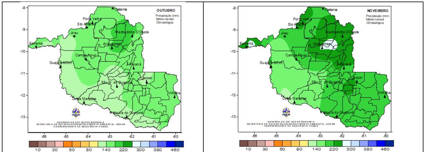
Fig. A- Climatologia de precipitação mensal , baseada no metodos dos Quantis - 1970 a 2011. Fonte: Atualização da base do ZSEE-RO.
