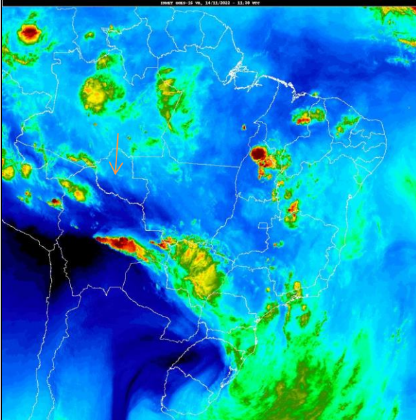
Fig. 1- Mapa da precipitação de 14/11/2022: Fonte: http://satellite.cptec.inpe.br/home/index.jsp
