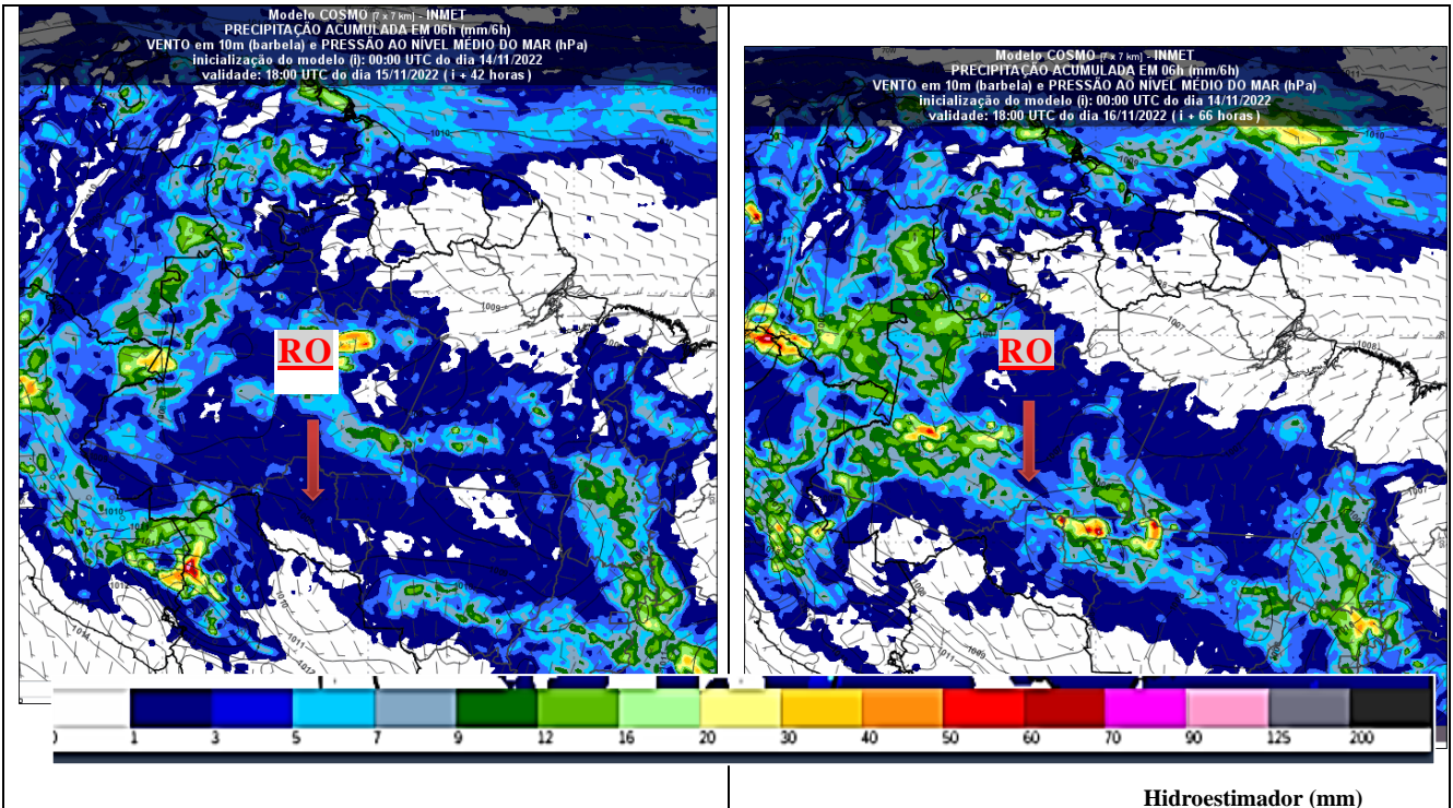
Figura 4 – Previsão de precipitação acumulada em RO, válida para 15/11/2022 18h Fonte: http://www.inmet.gov.br/
