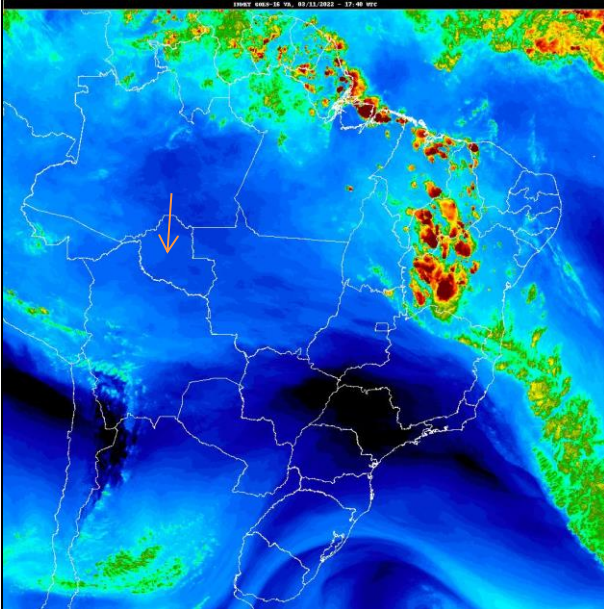
Fig. 1- Mapa da precipitação de 03/11/2022: Fonte: http://satelite.cptec.inpe.br/home/index.jsp
