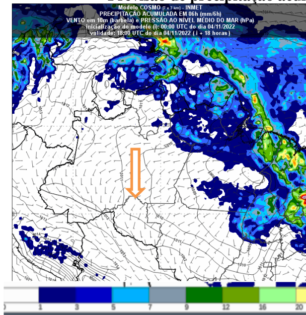
Figura 2 – Previsão do tempo no Estado de Rondônia para o dia 03/11/2022 as 18UTC
