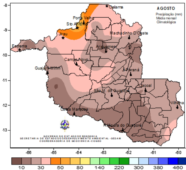
Figura 5 - Climatologia de precipitação mensal, baseada nos métodos dos Quantis - 1970 a 2011 (agosto)
