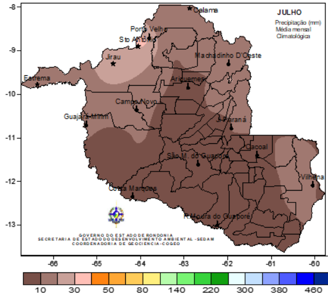
Figura 4 -. Climatologia de precipitação mensal , baseada no métodos dos Quantis - 1970 a 2011 (julho)
