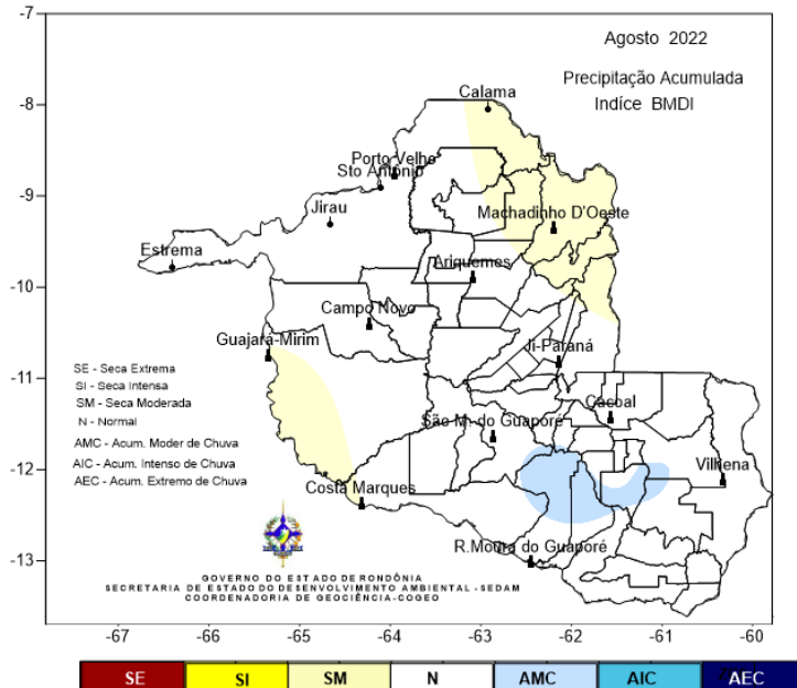
Figura 3 - Classificação da precipitação acumulada pelo Índice BMDI em agosto de 2022, com base nos dados do ZEE/RO, SEDAM/RO, ANA e INMET.
