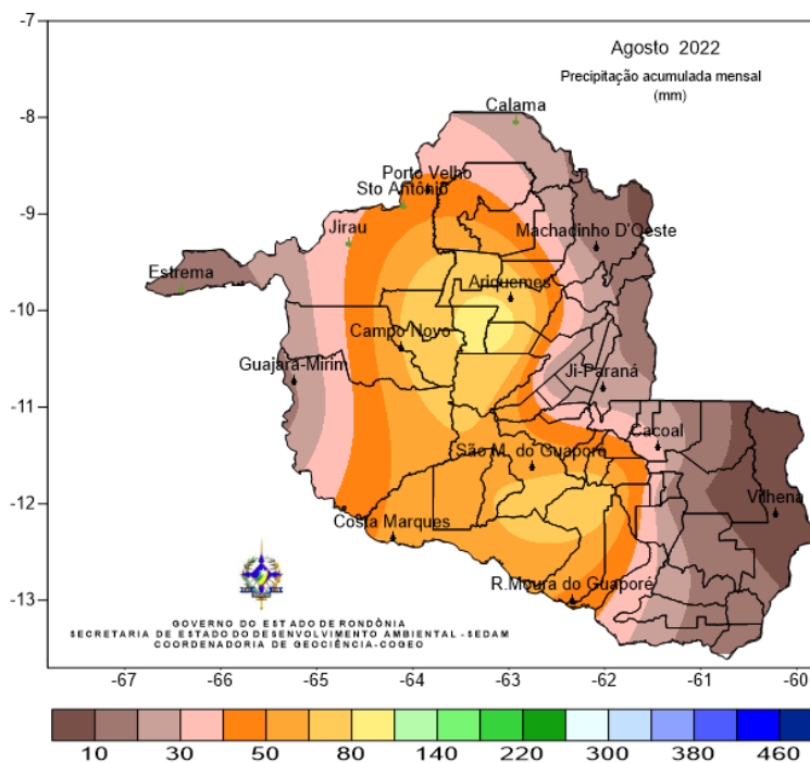
Figura 2 - Mapa da precipitação acumulada em agosto de 2022, com base nos dados da SEDAM/RO, ANA e INMET
