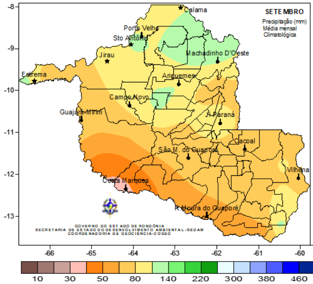
Figura 6 - Climatologia de precipitação mensal, baseada nos métodos dos Quantis - 1970 a 2011 (setembro)
