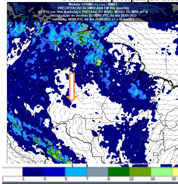
Figura 2 – Previsão do tempo no Estado de Rondônia para o dia 26/09/2022 as 18UTC
