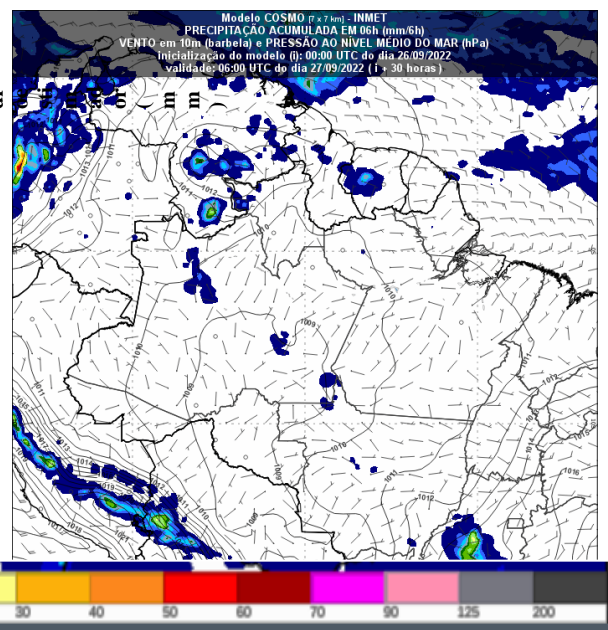
Figura 3 – Previsão do tempo no Estado de Rondônia para o dia 27/09/2022 as 06 UTC
