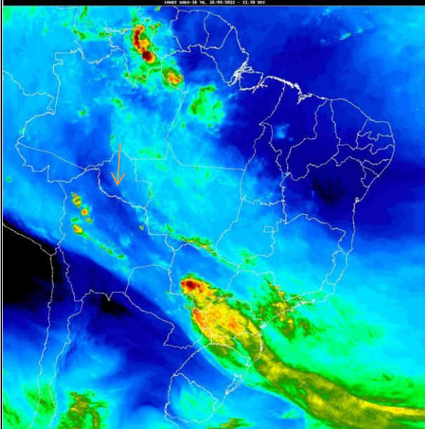
Fig. 1- Mapa da precipitação de 26/09/2022: Fonte: http://satellite.cptec.inpe.br/home/index.jsp
