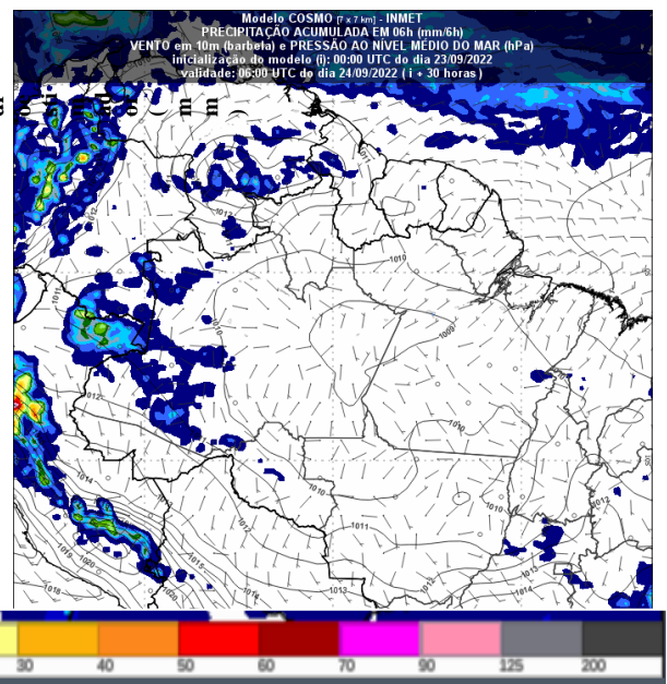
Figura 3 – Previsão do tempo no Estado de Rondônia para o dia 24/09/2022 as 06 UTC
