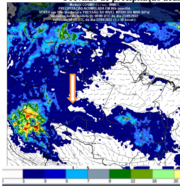
Figura 2 – Previsão do tempo no Estado de Rondônia para o dia 23/09/2022 as 18UTC
