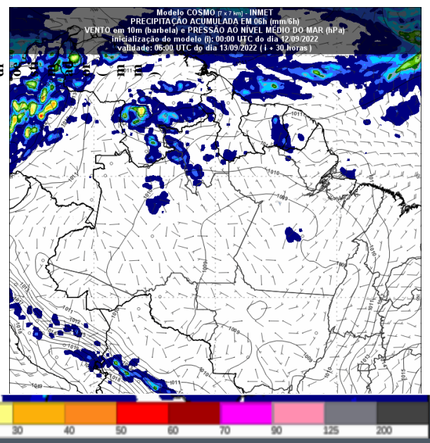
Figura 3 – Previsão do tempo no Estado de Rondônia para o dia 13/09/2022 as 06 UTC
