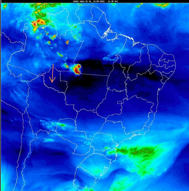
Fig. 1- Mapa da precipitação de 12/09/2022: Fonte: http://satellite.cptec.inpe.br/home/index.jsp
