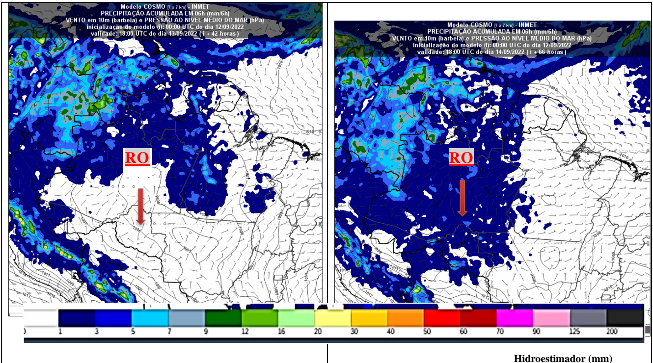
Figura 4 – Previsão de precipitação acumulada em RO, válida para 13/09/2022 18h Fonte: http://www.inmet.gov.br/
