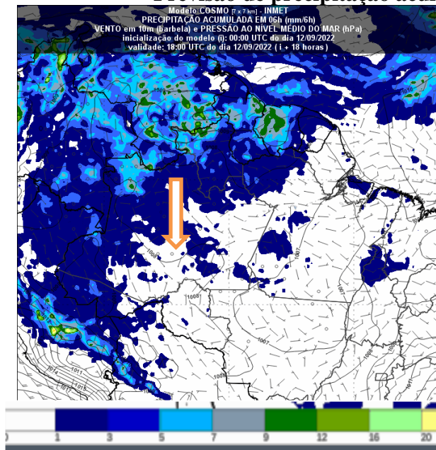
Figura 2 – Previsão do tempo no Estado de Rondônia para o dia 12/09/2022 as 18UTC
