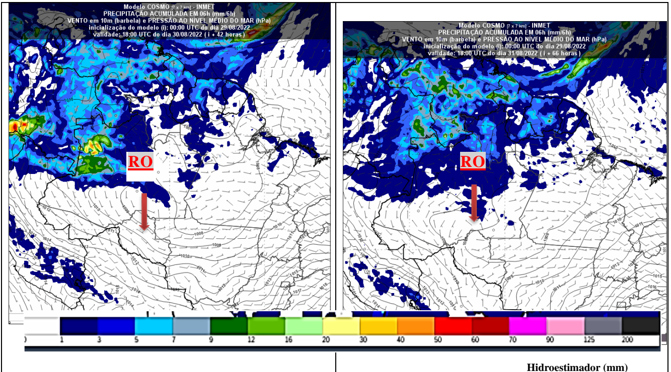
Figura 4 – Previsão de precipitação acumulada em RO, válida para 30/08/2022 18h Fonte: http://www.inmet.gov.br/
