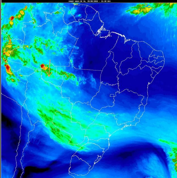
Fig. 1- Mapa da precipitação de 29/08/2022: Fonte: http://satellite.cptec.inpe.br/home/index.jsp
