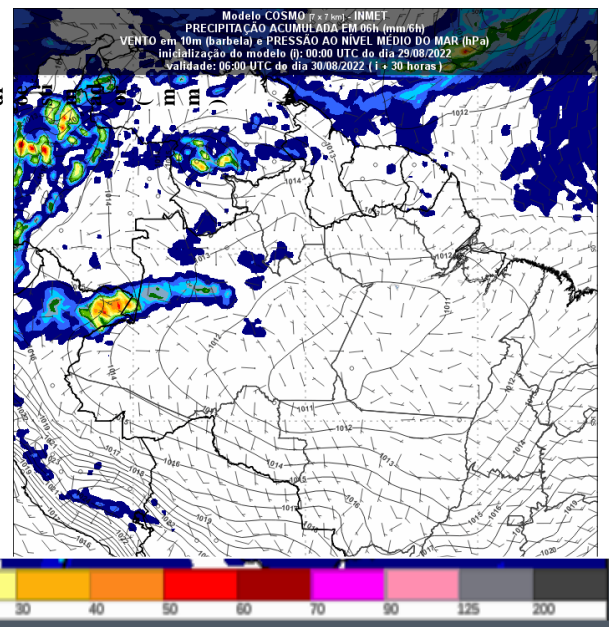
Figura 3 – Previsão do tempo no Estado de Rondônia para o dia 30/08/2022 as 06 UTC
