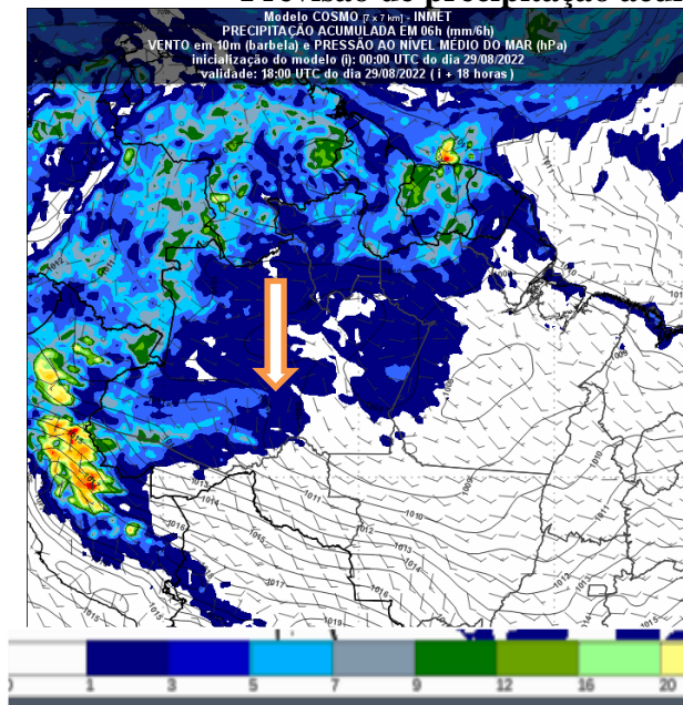
Figura 2 – Previsão do tempo no Estado de Rondônia para o dia 29/08/2022 as 18UTC
