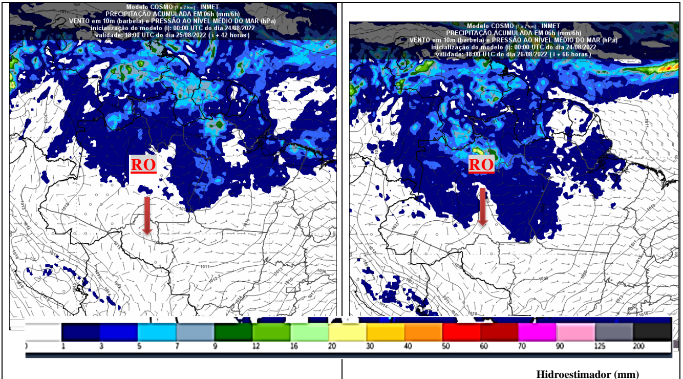
Figura 4 – Previsão de precipitação acumulada em RO, válida para 25/08/2022 18h Fonte: http://www.inmet.gov.br/
