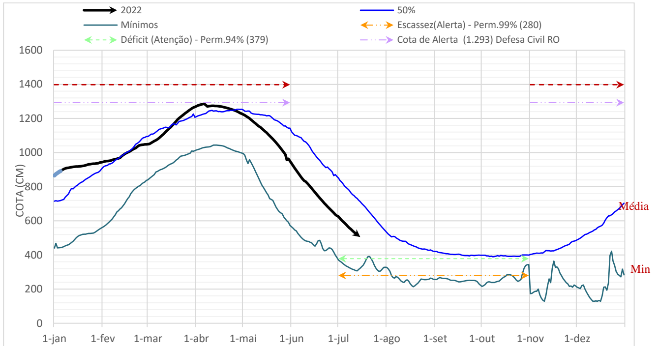
Gráfico 1- Monitoramento diário da cota do rio Guaporé, na coordenada geográfica de latitude 12,4267°leste e longitude 64,4253° oeste, município de Costa Marques/RO - Série histórica 1968 a 2017.
