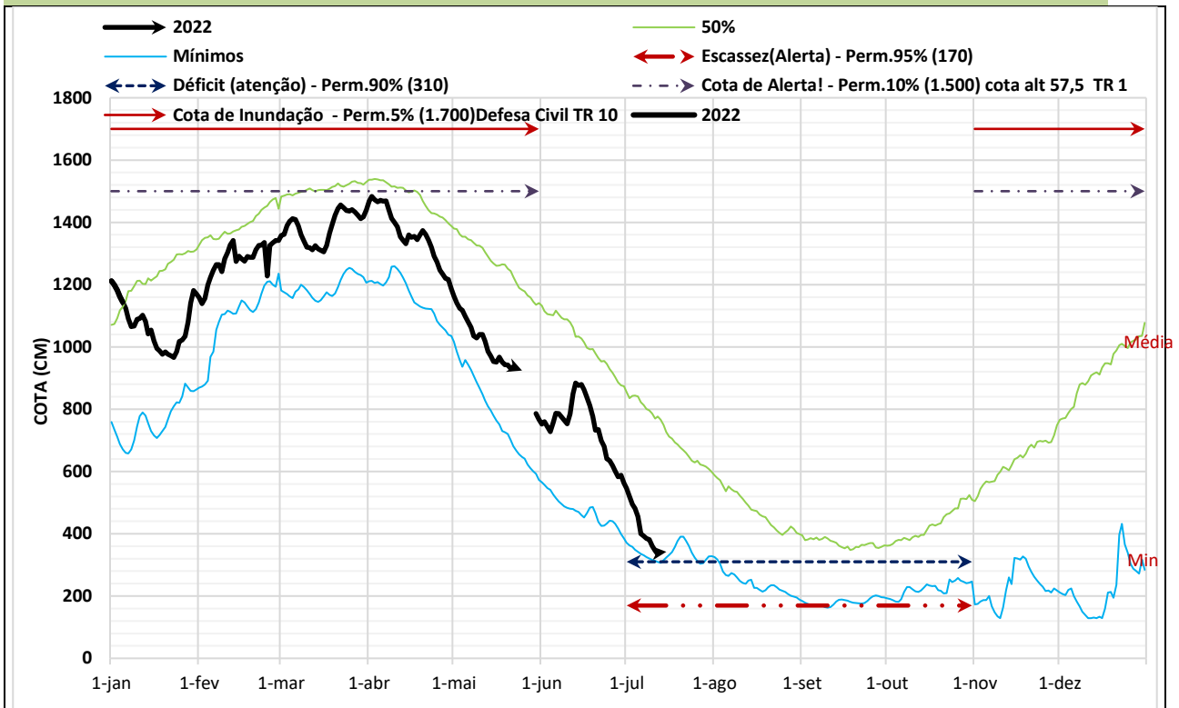
Gráfico 3 - Monitoramento diário da cota do rio Madeira, na coordenada geográfica de latitude -8,7483 leste e longitude -63,9169 c. Ponte Br-319, Porto Velho/RO.
