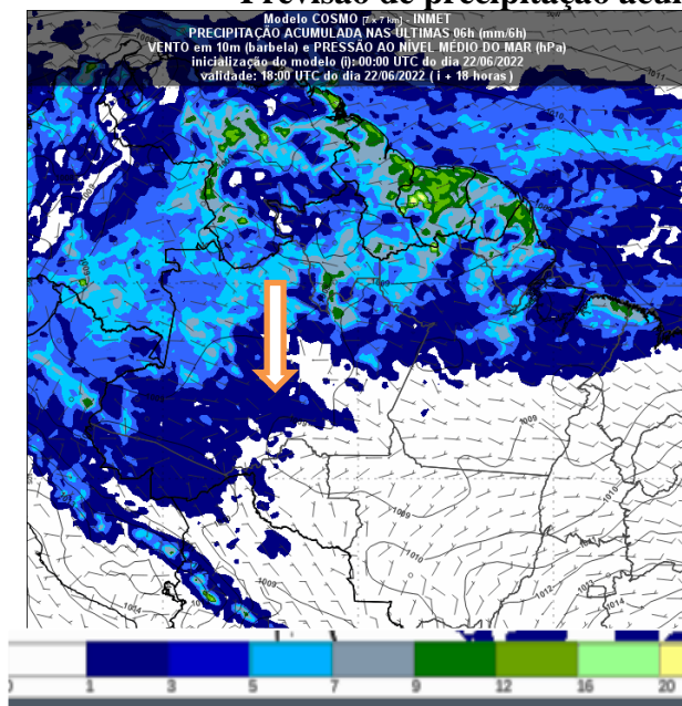
Figura 2 – Previsão do tempo no Estado de Rondônia para o dia 22/06/2022 as 18UTC
