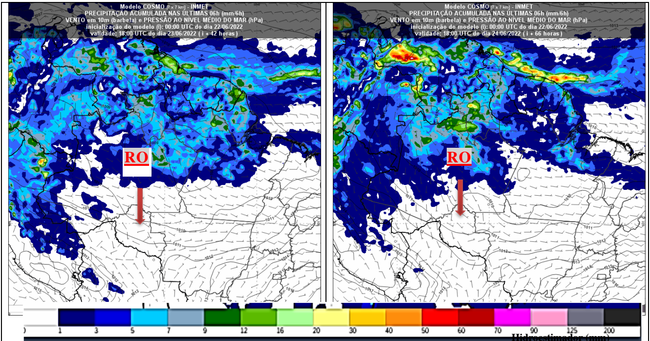
Figura 4 – Previsão de precipitação acumulada em RO, válida para 23/06/2022 18h Fonte: http://www.inmet.gov.br/
