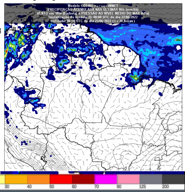
Figura 3 – Previsão do tempo no Estado de Rondônia para o dia 23/06/2022 as 06 UTC
