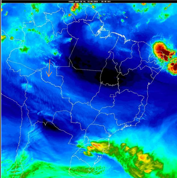
Fig. 1- Mapa da precipitação de 22/06/2022: Fonte: http://satellite.cptec.inpe.br/home/index.jsp
