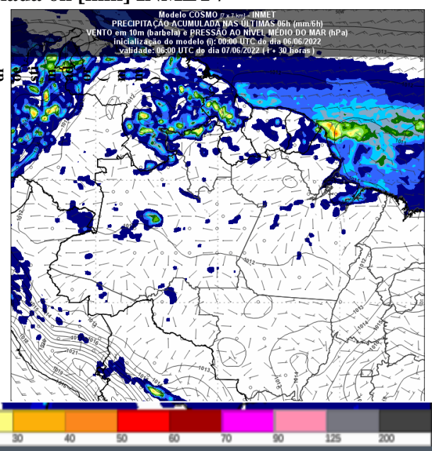
Figura 3 – Previsão do tempo no Estado de Rondônia para o dia 07/06/2022 as 06 UTC
