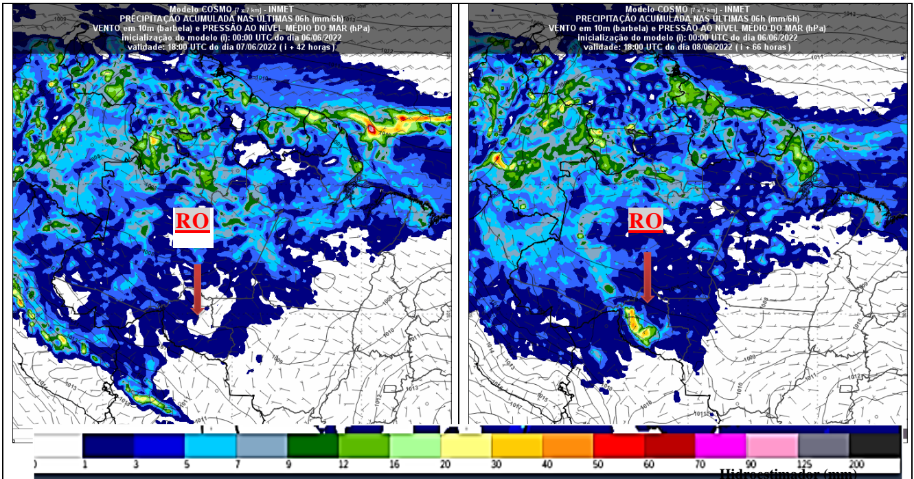
Figura 4 – Previsão de precipitação acumulada em RO, válida para 07/06/2022 18h Fonte: http://www.inmet.gov.br/
