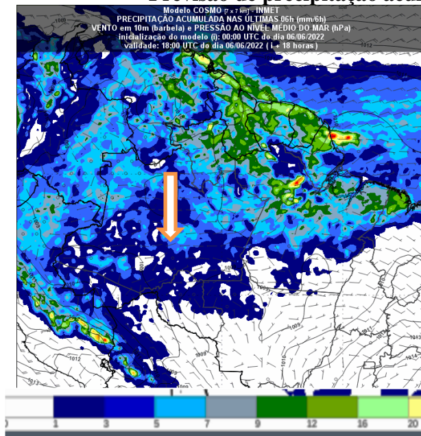
Figura 2 – Previsão do tempo no Estado de Rondônia para o dia 06/06/2022 as 18UTC
