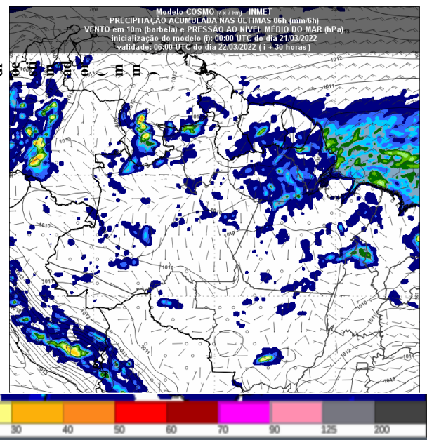
Figura 3 – Previsão do tempo no Estado de Rondônia para o dia 22/03/2022 as 06 UTC
