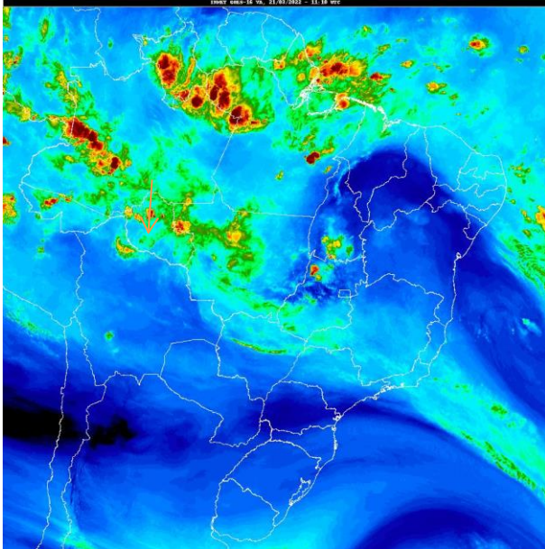
Fig. 1- Mapa da precipitação de 21/03/2022: Fonte: http://satellite.cptec.inpe.br/home/index.jsp
