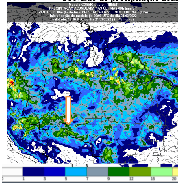
Figura 2 – Previsão do tempo no Estado de Rondônia para o dia 21/03/2022 as 18UTC
