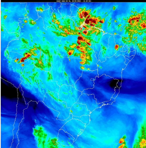
Fig. 1- Mapa da precipitação de 18/03/2022: Fonte: http://satellite.cptec.inpe.br/home/index.jsp
