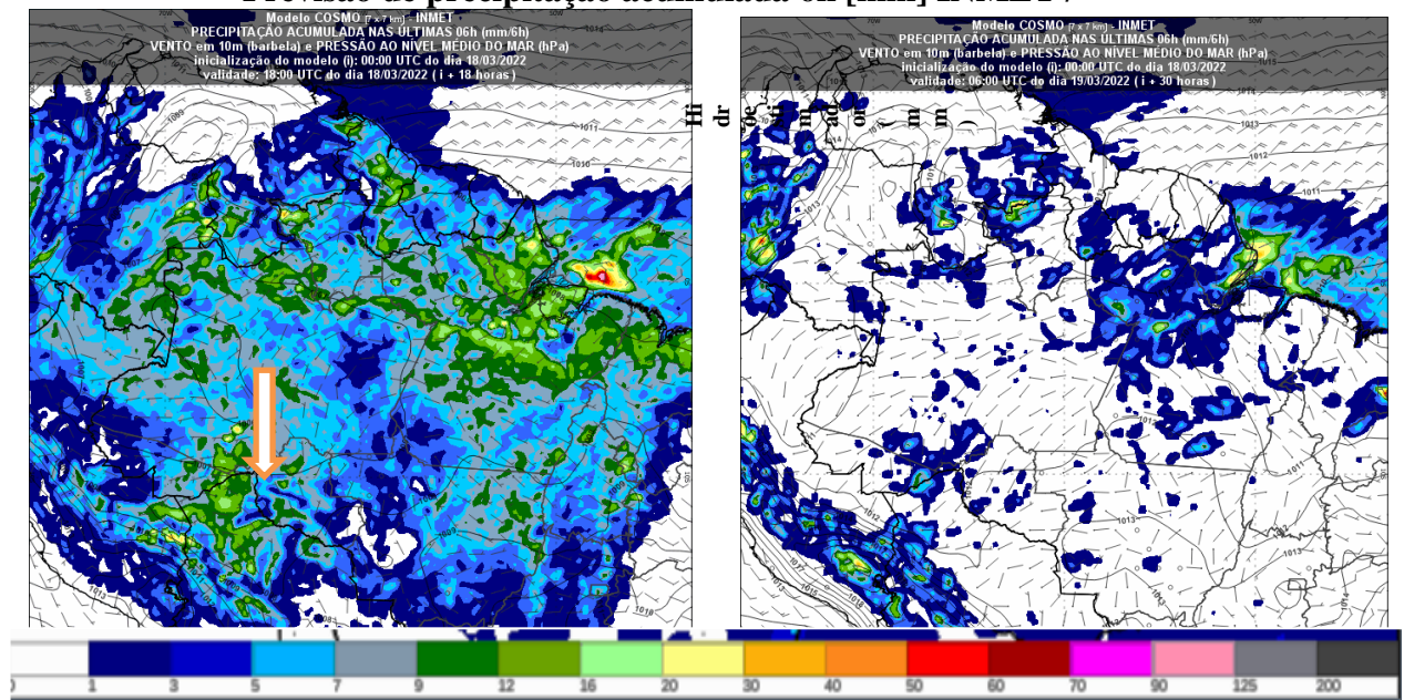
Figura 2 – Previsão do tempo no Estado de Rondônia para o dia 18/03/2022 as 18UTC
