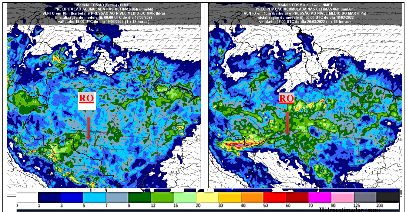
Figura 4 – Previsão de precipitação acumulada em RO, válida para 19/03/2022 18h
