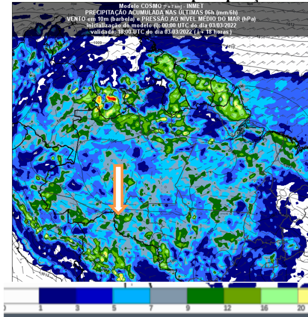
Figura 2 – Previsão do tempo no Estado de Rondônia para o dia 03/03/2022 as 18UTC
