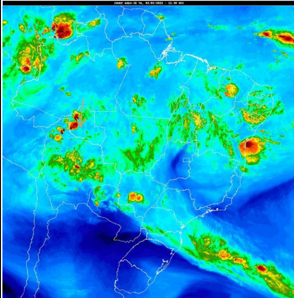
Fig. 1- Mapa da precipitação de 03/03/2022: Fonte: http://satelite.cptec.inpe.br/home/index.jsp
