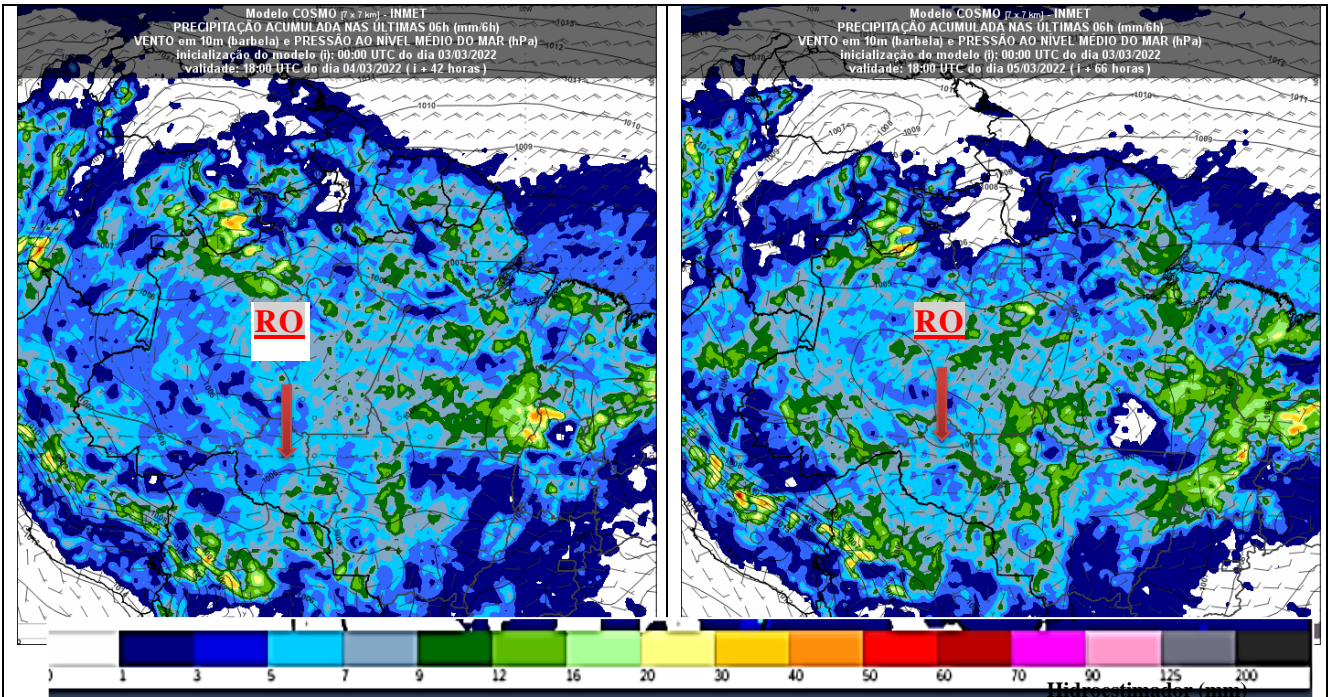
Figura 4 – Previsão de precipitação acumulada em RO, válida para 04/03/2022 18h Fonte: http://www.inmet.gov.br/
