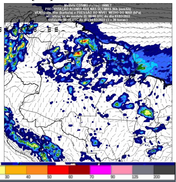
Figura 3 – Previsão do tempo no Estado de Rondônia para o dia 04/03/2022 as 06 UTC
