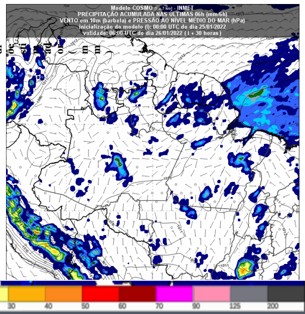
Figura 3 – Previsão do tempo no Estado de Rondônia para o dia 26/01/2022 as 06 UTC
