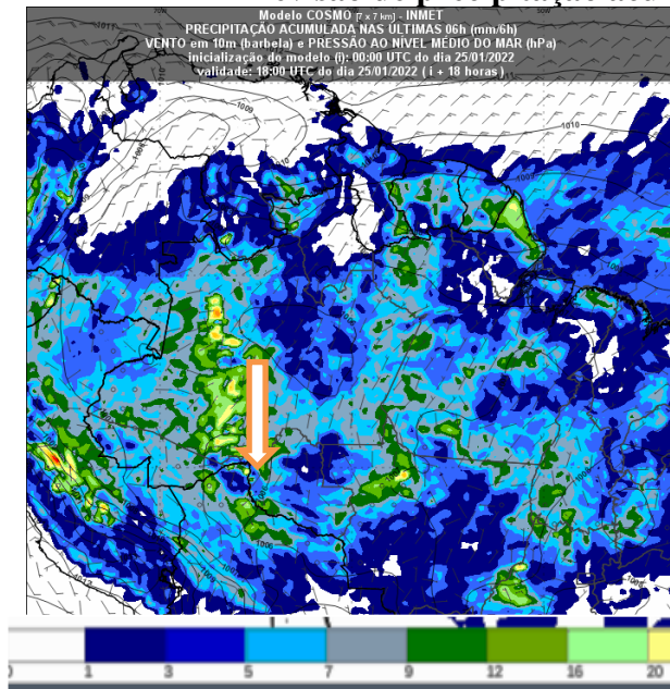
Figura 2 – Previsão do tempo no Estado de Rondônia para o dia 25/01/2022 as 18UTC
