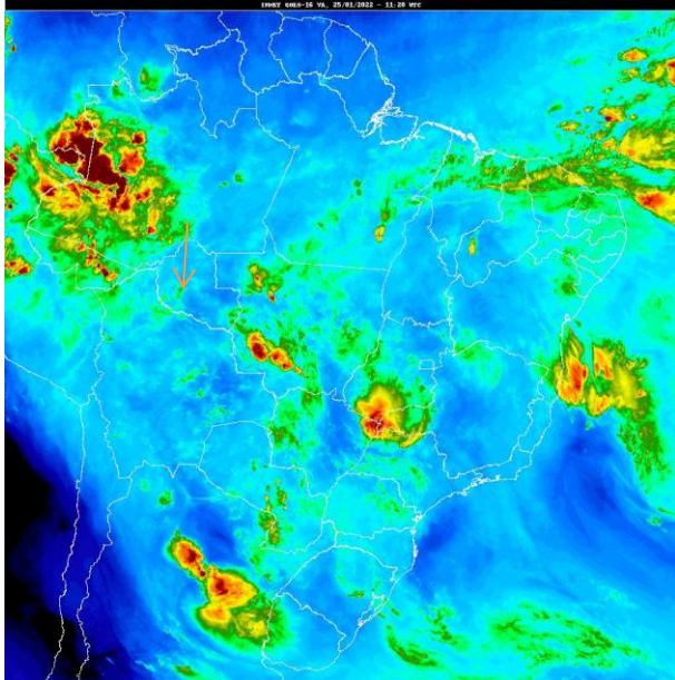
Fig. 1- Mapa da precipitação de 25/01/2022: Fonte: http://satellite.cptec.inpe.br/home/index.jsp
