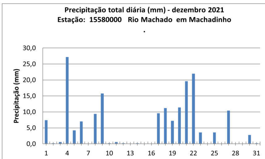
Gráfico 1 - Monitoramento da precipitação total diária, com base nos dados da estação pluviométrica do Rio Machado no município de Machadinho - código estação Hidrometeorológica de Tabajara 15580000
