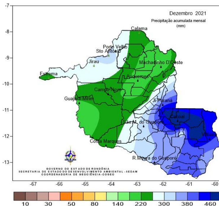
Figura 2 - Mapa da precipitação acumulada em dezembro de 2021, com base nos dados da SEDAM/RO, ANA e INMET
