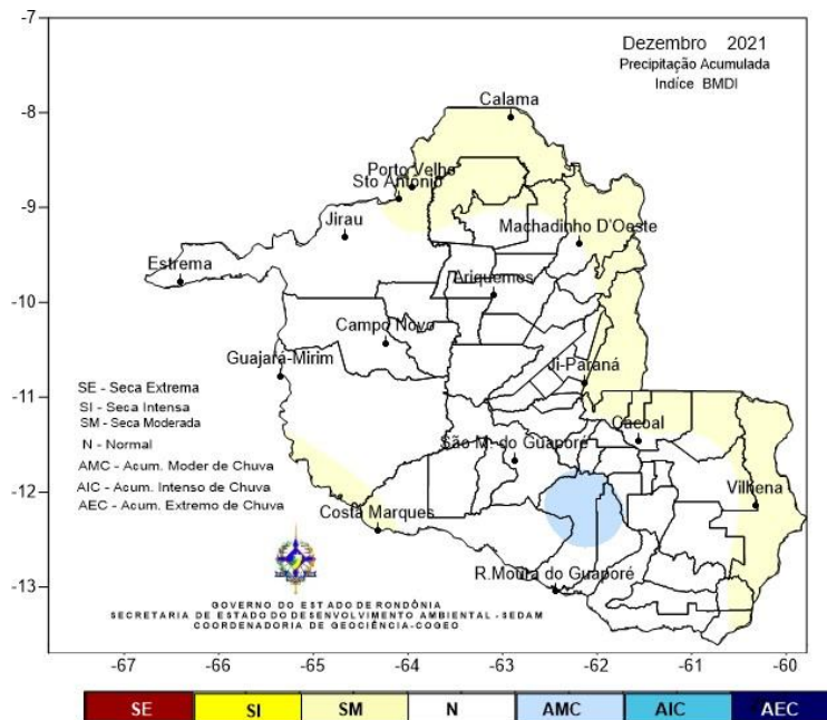
Figura 3 - Classificação da precipitação acumulada pelo Índice BMDI em dezembro de 2021, com base nos dados do ZEE/RO, SEDAM/RO, ANA e INMET.
