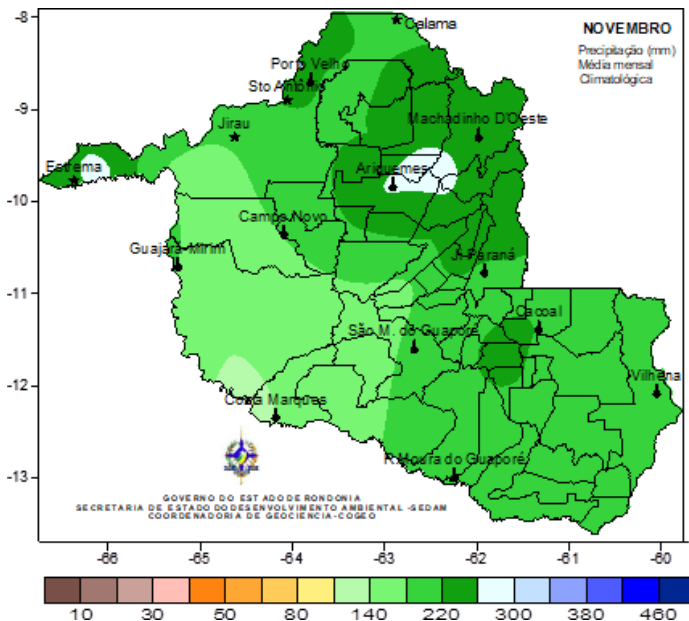
Figura 4 -. Climatologia de precipitação mensal , baseada no metodos dos Quantis - 1970 a 2011 (novembro)
