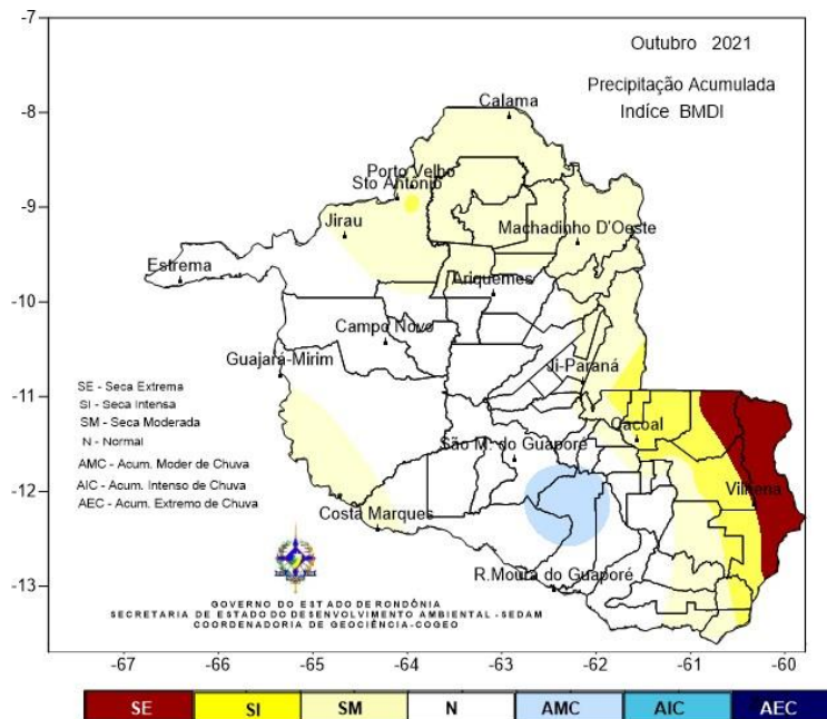
Figura 3 - Classificação da precipitação acumulada pelo Índice BMDI em outubro de 2021, com base nos dados do ZEE/RO, SEDAM/RO, ANA e INMET.
