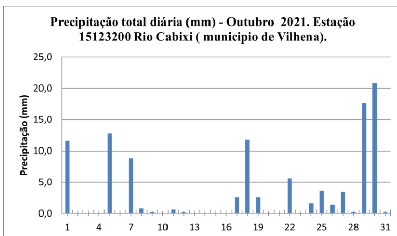
Gráfico 1 - Monitoramento da precipitação total diária, com base nos dados da estação pluviométrica do Rio Cabixi no município de Vilhena - código estação Hidrometeorológica 15123200
