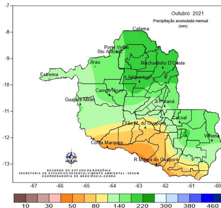
Figura 2 - Mapa da precipitação acumulada em outubro de 2021, com base nos dados da SEDAM/RO, ANA e INMET
