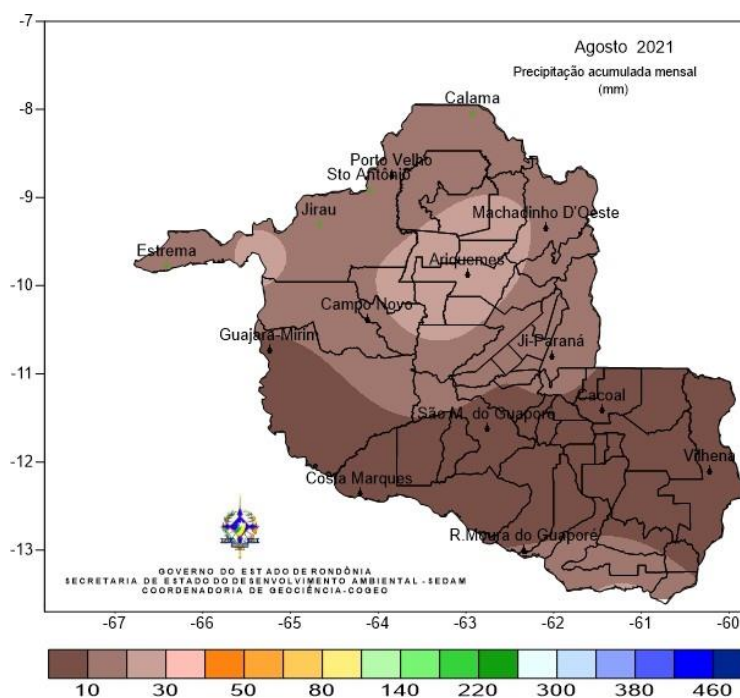
Figura 2 - Mapa da precipitação acumulada em agosto de 2021, com base nos dados da SEDAM/RO, ANA e INMET
