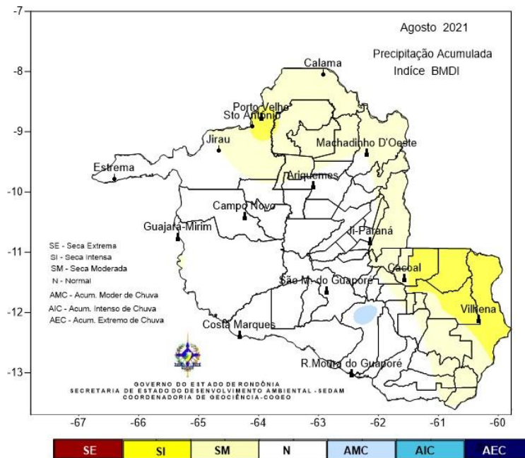
Figura 3 - Classificação da precipitação acumulada pelo Índice BMDI em agosto de 2021, com base nos dados do ZEE/RO, SEDAM/RO, ANA e INMET.
