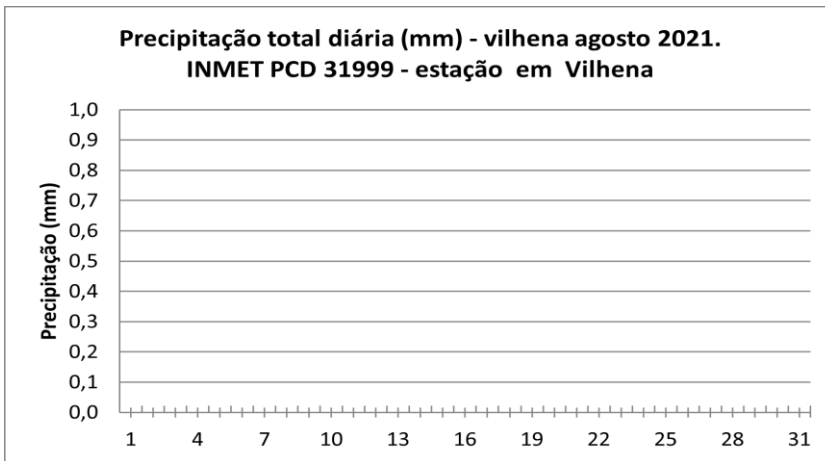
Gráfico 2 - Precipitação total diária estação meteorológica no município de Vilhena
