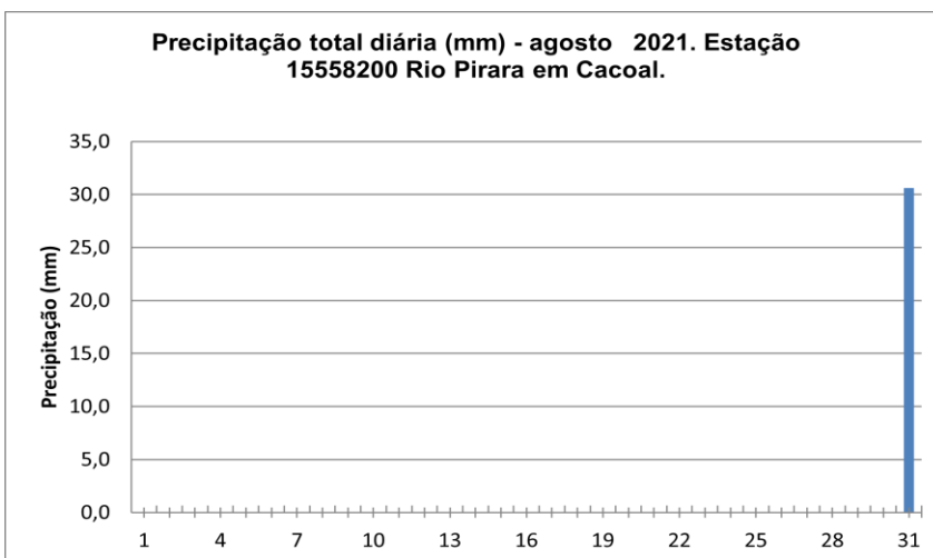
Gráfico 3 - Precipitação total diária estação Hidrometeorológica de Cacoal localizada na Bacia do Rio Machado.
